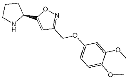
5 10 (S)-3-((3,4-Dimethoxyphenoxy)methyl)-5-(pyrrolidin-2-yl)isoxazole
