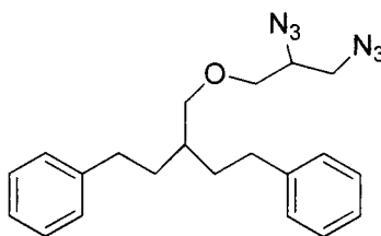
(3-((2,3-diazidopropoxy)methyl)pentane-1,5-diyl)dibenzene
