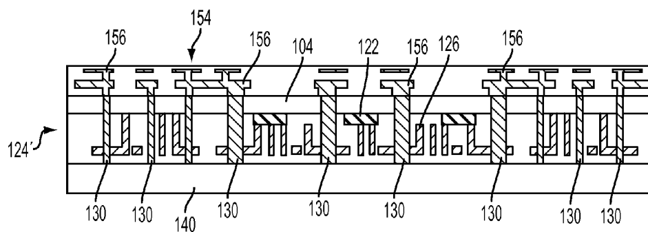
FIG. 9D
