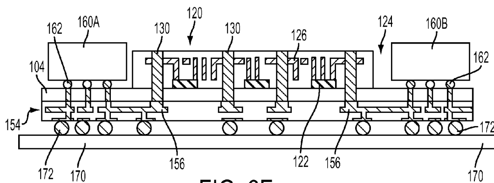
FIG. 6F
