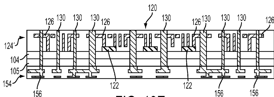
FIG. 10E
