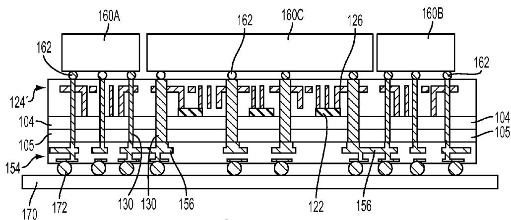
FIG. 10F
