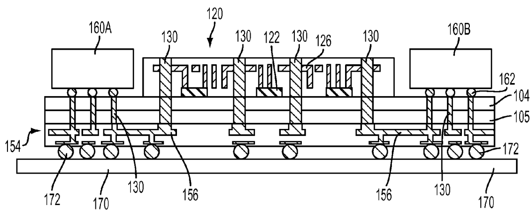
FIG. 7F
