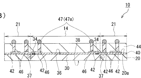
この発明の半導体装置を示す図(2)
