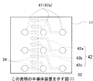
この発明の半導体装置を示す図(1)
