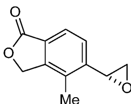
4-methyl-5-[(2R)-oxiran-2-yl]-2-benzofuran-1(3H)-one
