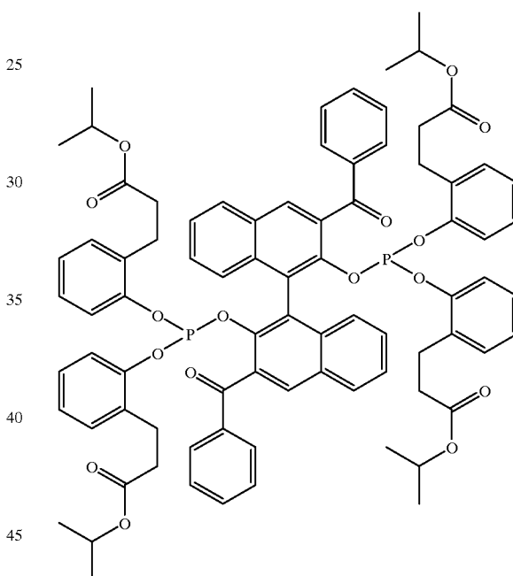
Ligand 4
