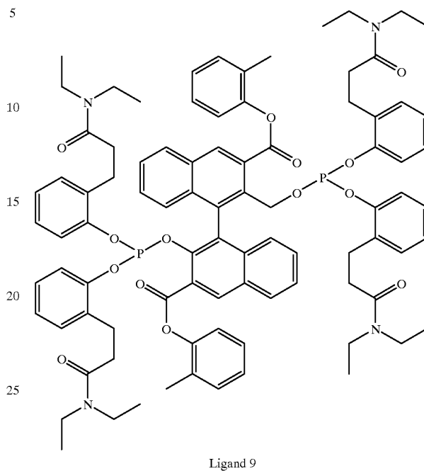
Ligand 9
