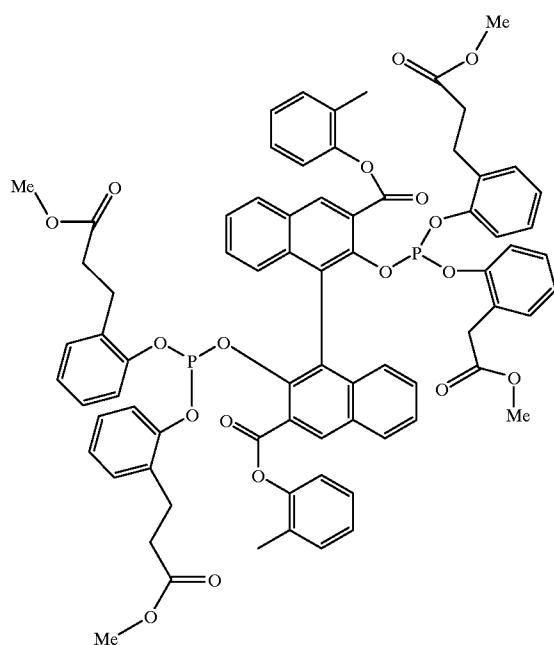
Ligand 3
