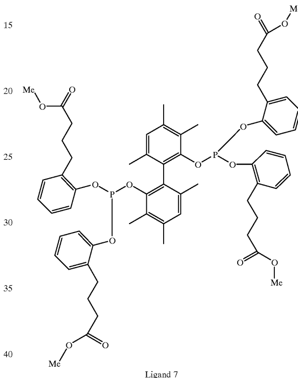
Ligand 7
