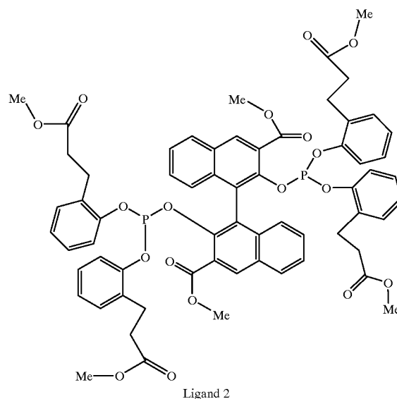
Ligand 2
