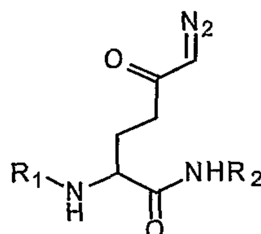
diazoketones
