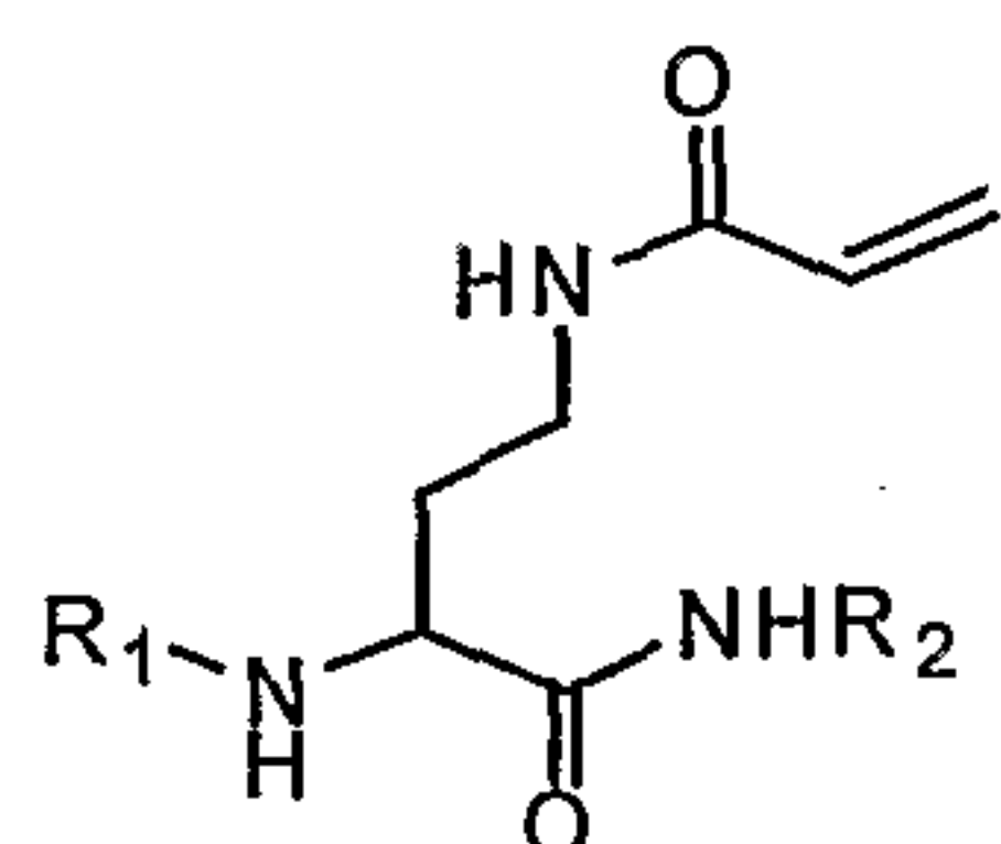
vinylogous amides
