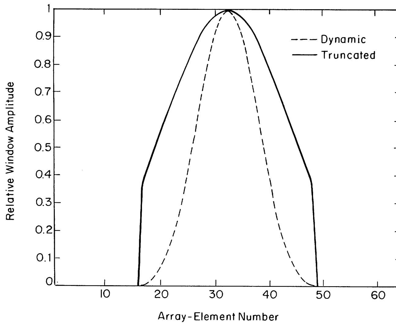
FIG. 28
