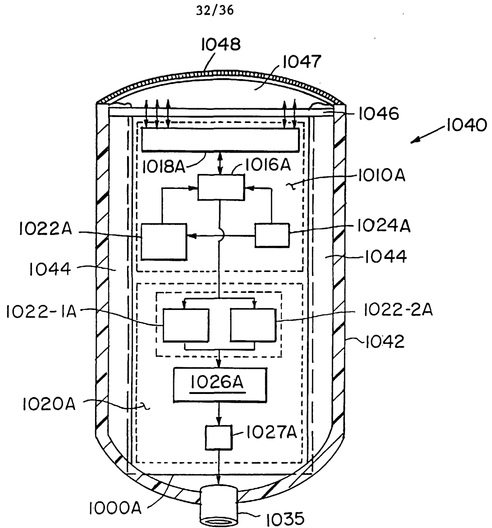
FIG. 34
