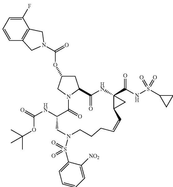
I-45
