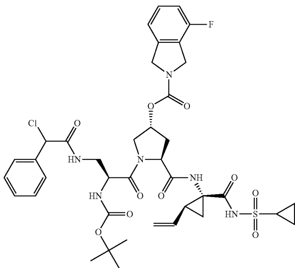
I-3
