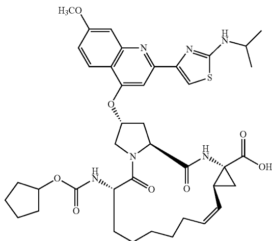
BILN 2061
