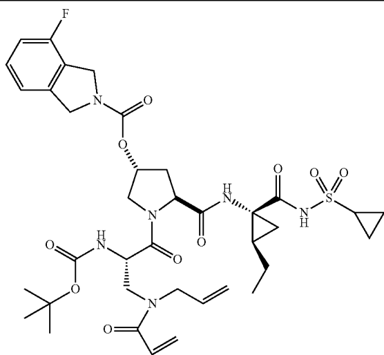
I-16
