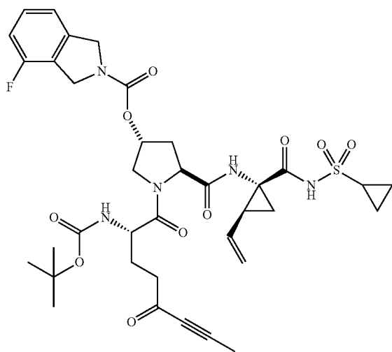
I-28
