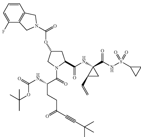
I-29
