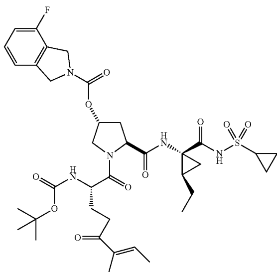
I-39
