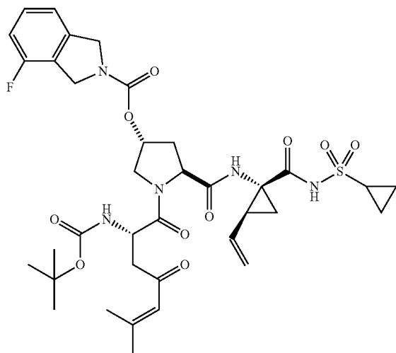
I-32
