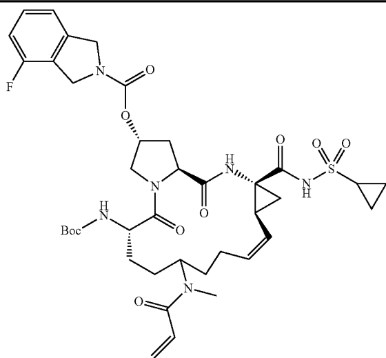
I-57
