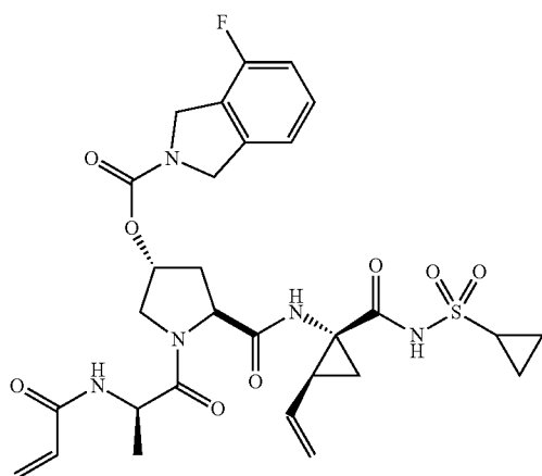
I-8
