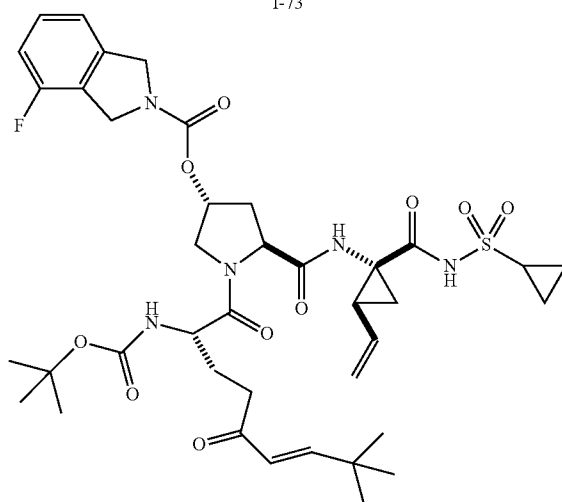
I-74
