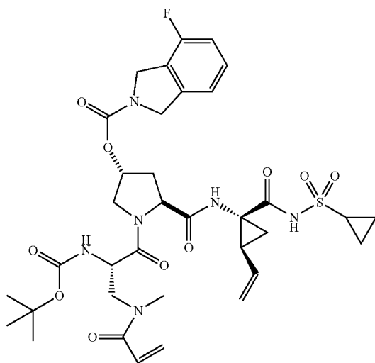
I-11
