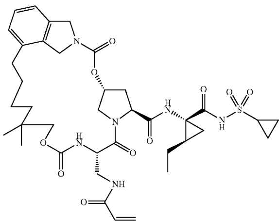
I-43
