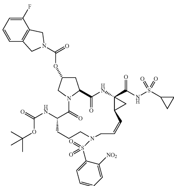
I-54
