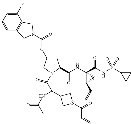
I-46
