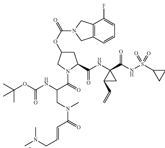
I-50
