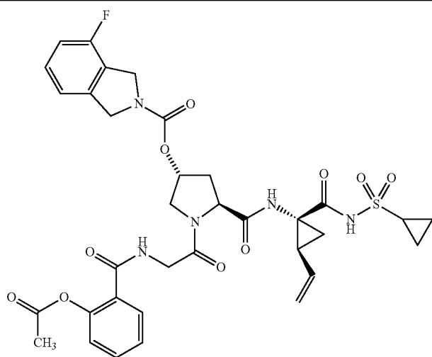
I-10
