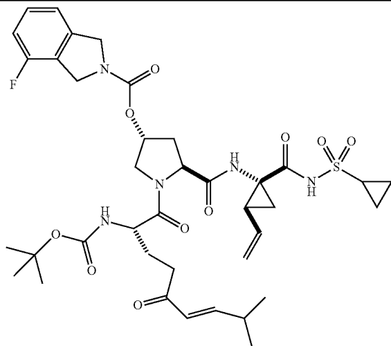
I-76
