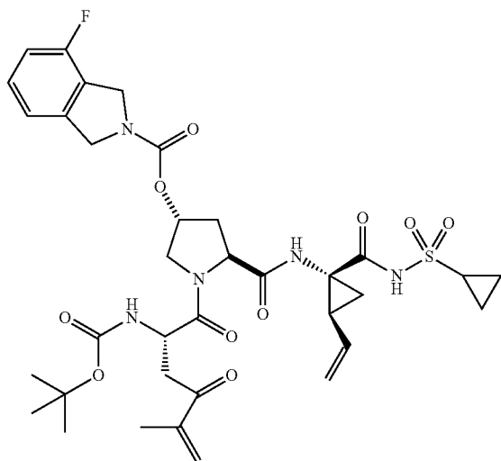
I-68
