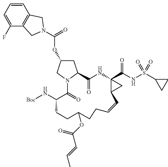
I-66
