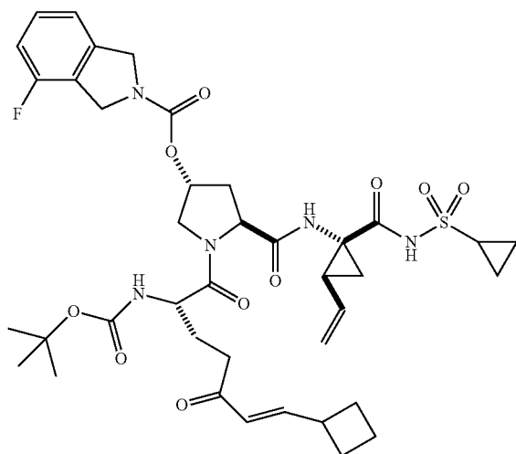
I-78
