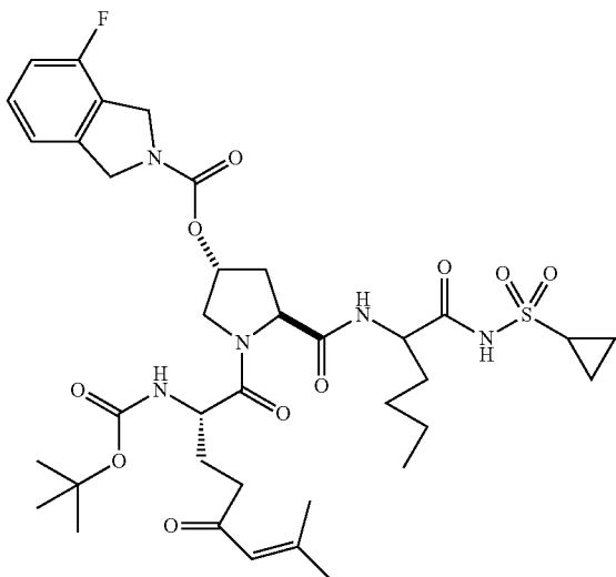
I-44
