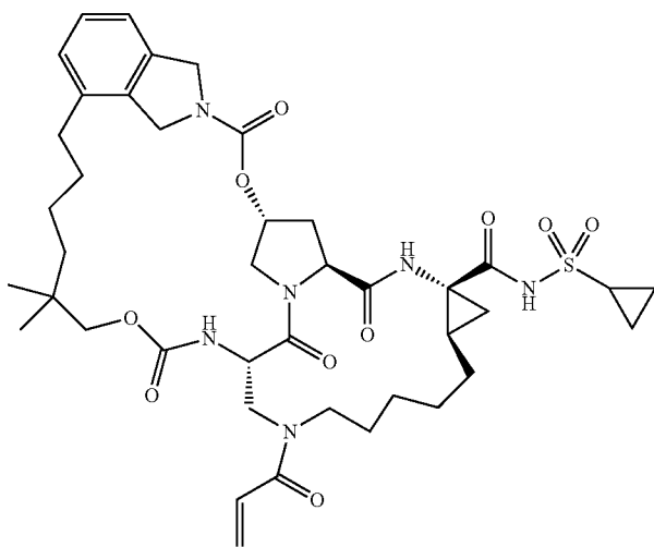
I-59
