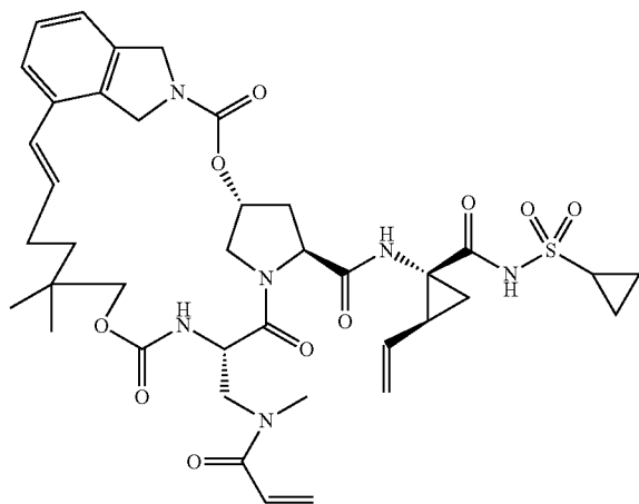
I-41
