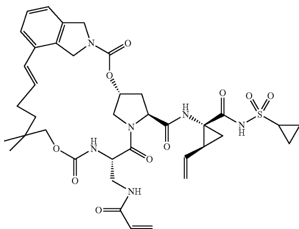
I-40
