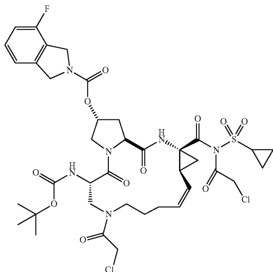
I-48
