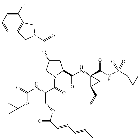
I-67
