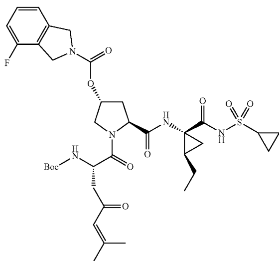
I-60
