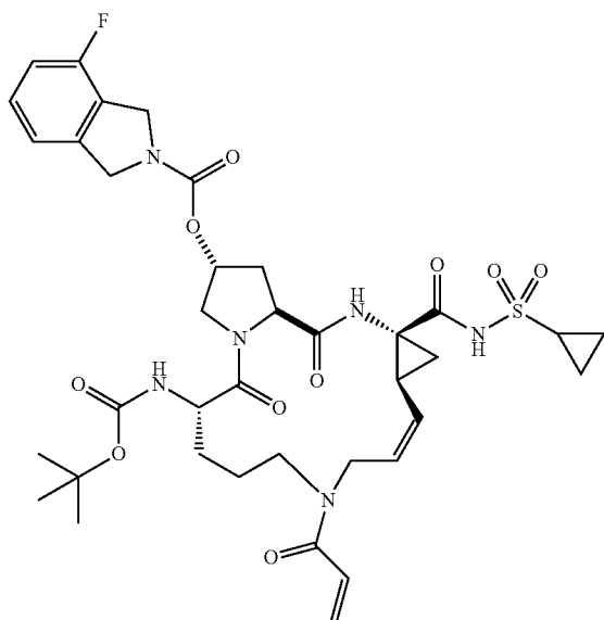
I-37
