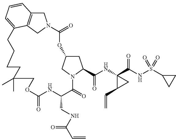
I-42
