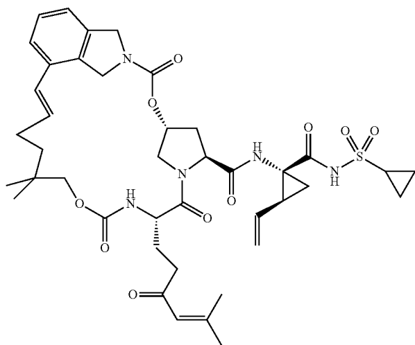
I-55
