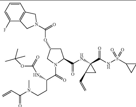
I-13
