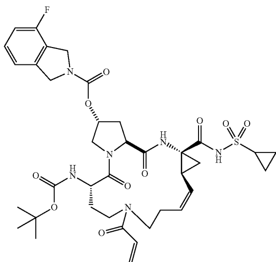
I-36
