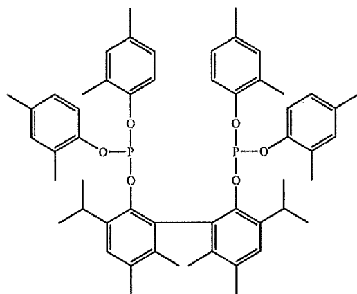
Ligand (V).
