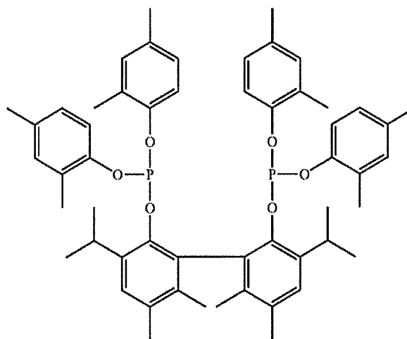
Ligand (V).
