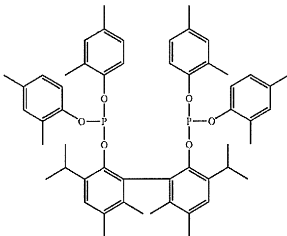
Ligand (V).
