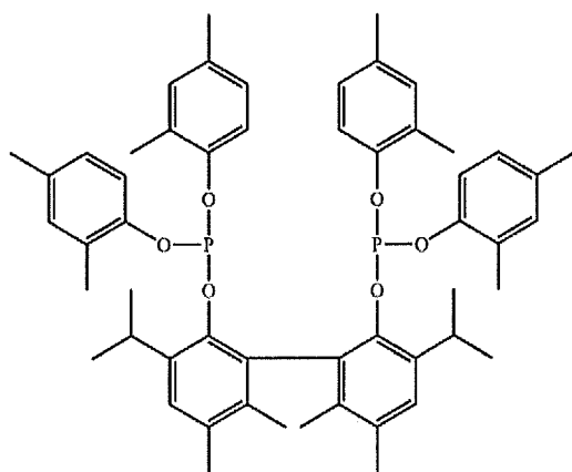
Ligand (V).
