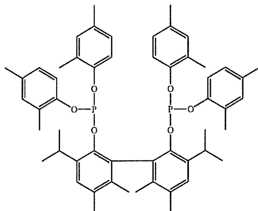
Ligand (V).
