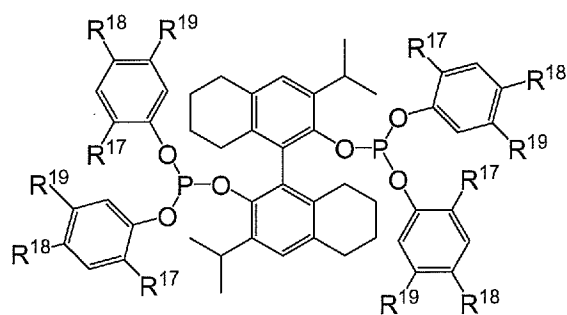
(VI)
