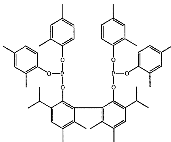
Ligand (V).
