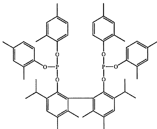
Ligand (V).
