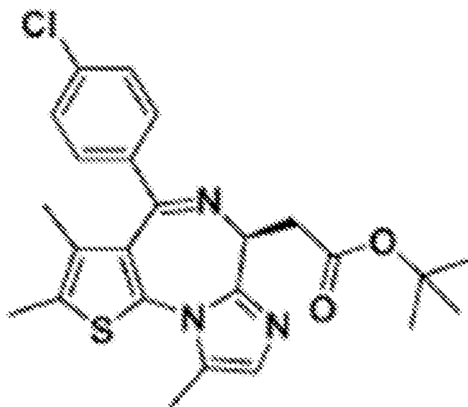
(VIII)
