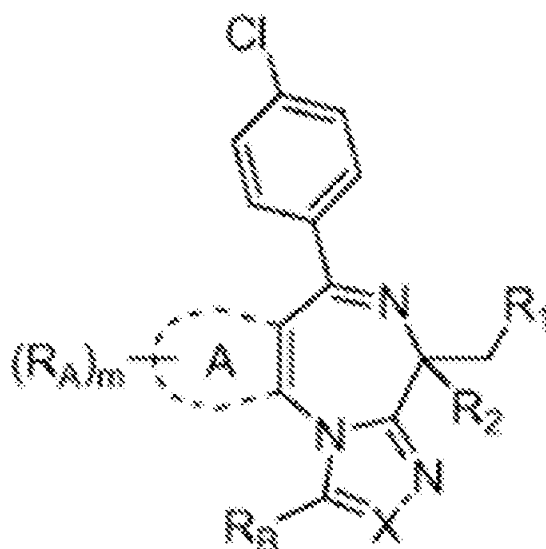
(IV)
