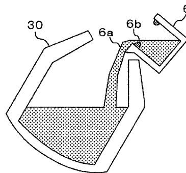
(CONVERTER POURING PROCESS)
