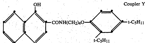
Coupler Y
