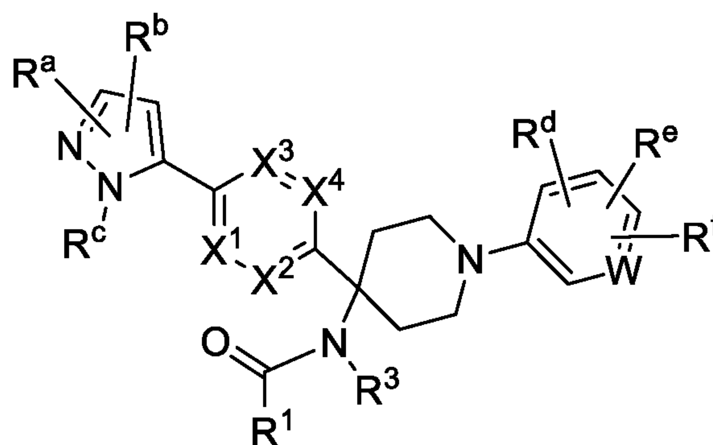
Formula (Vm)
