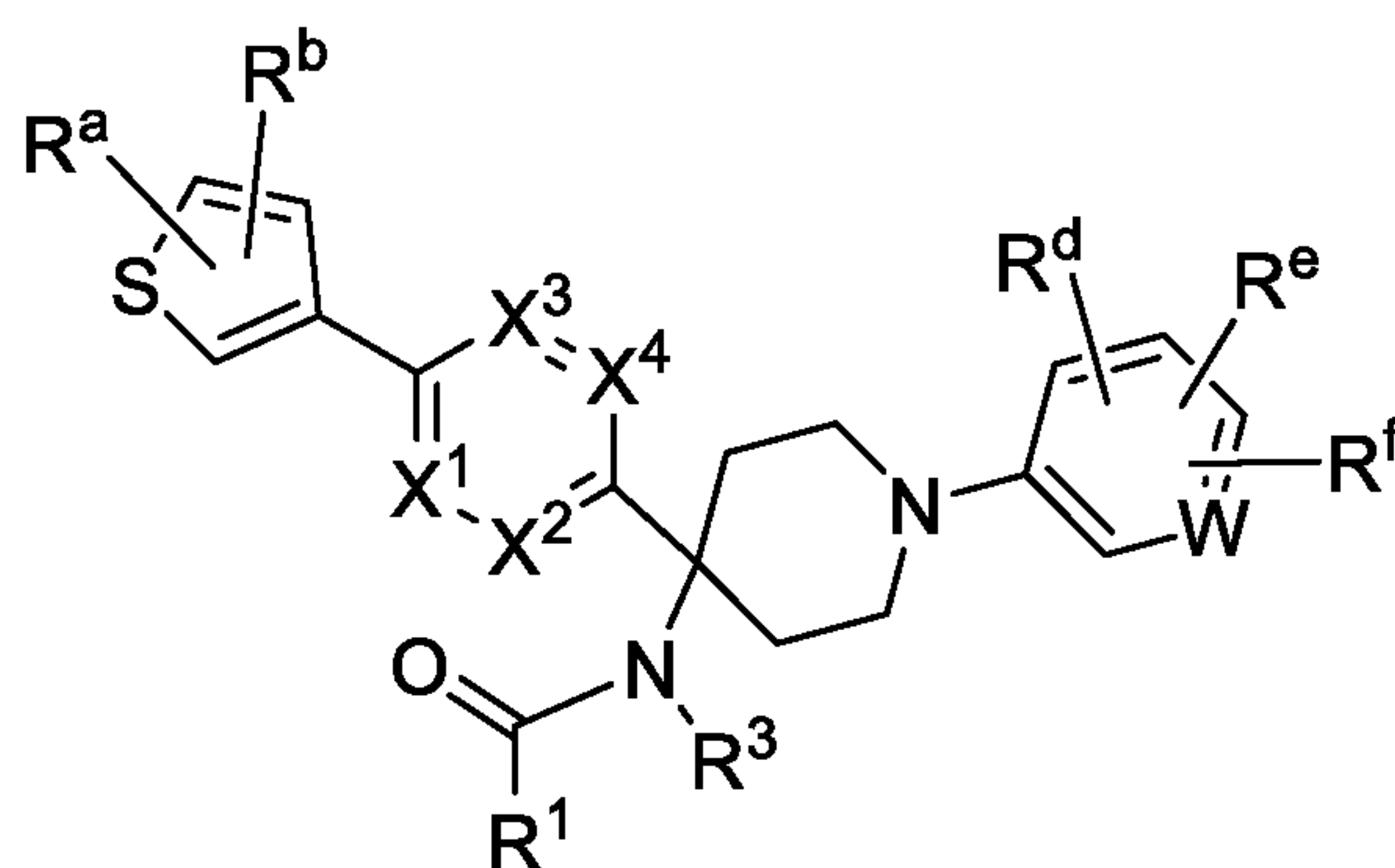
Formula (Vo)
