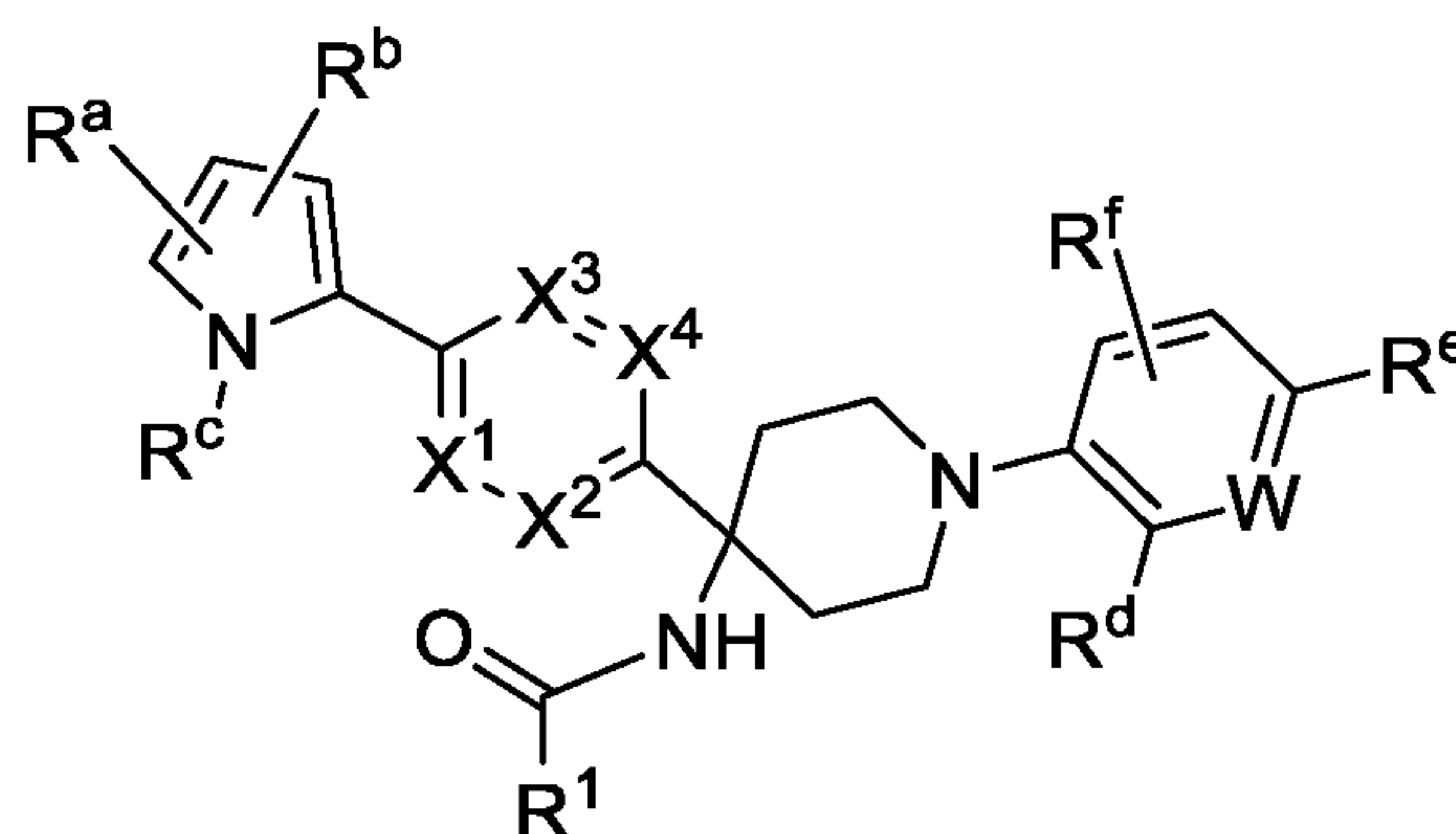
Formula (VIId)
