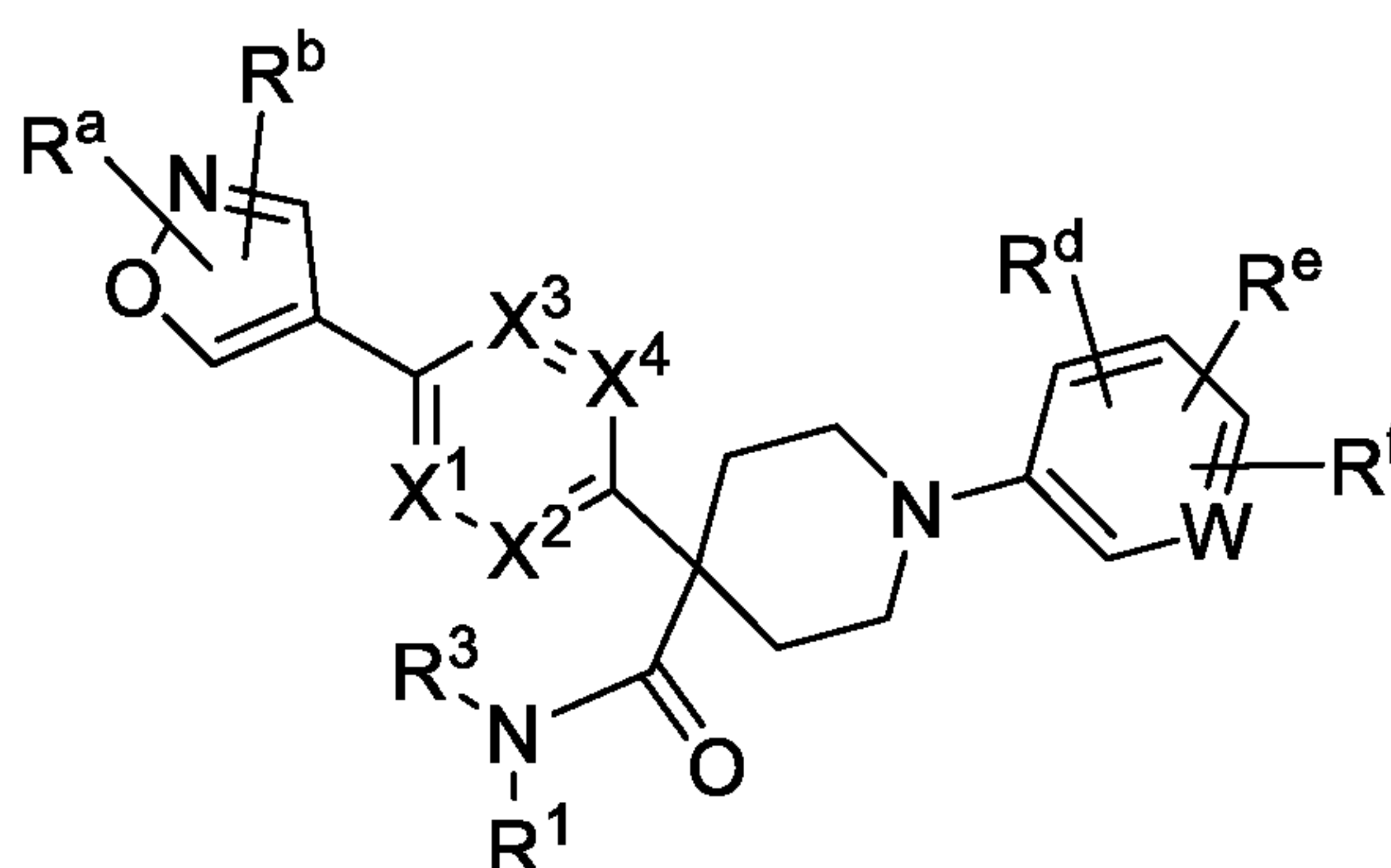
Formula (Vf)
