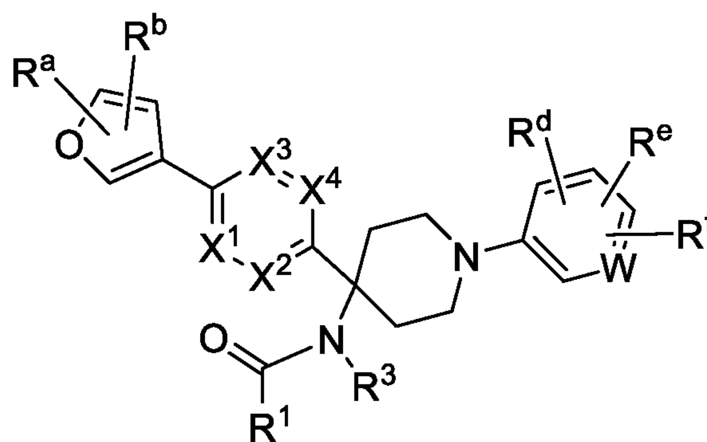
Formula (Vo)
