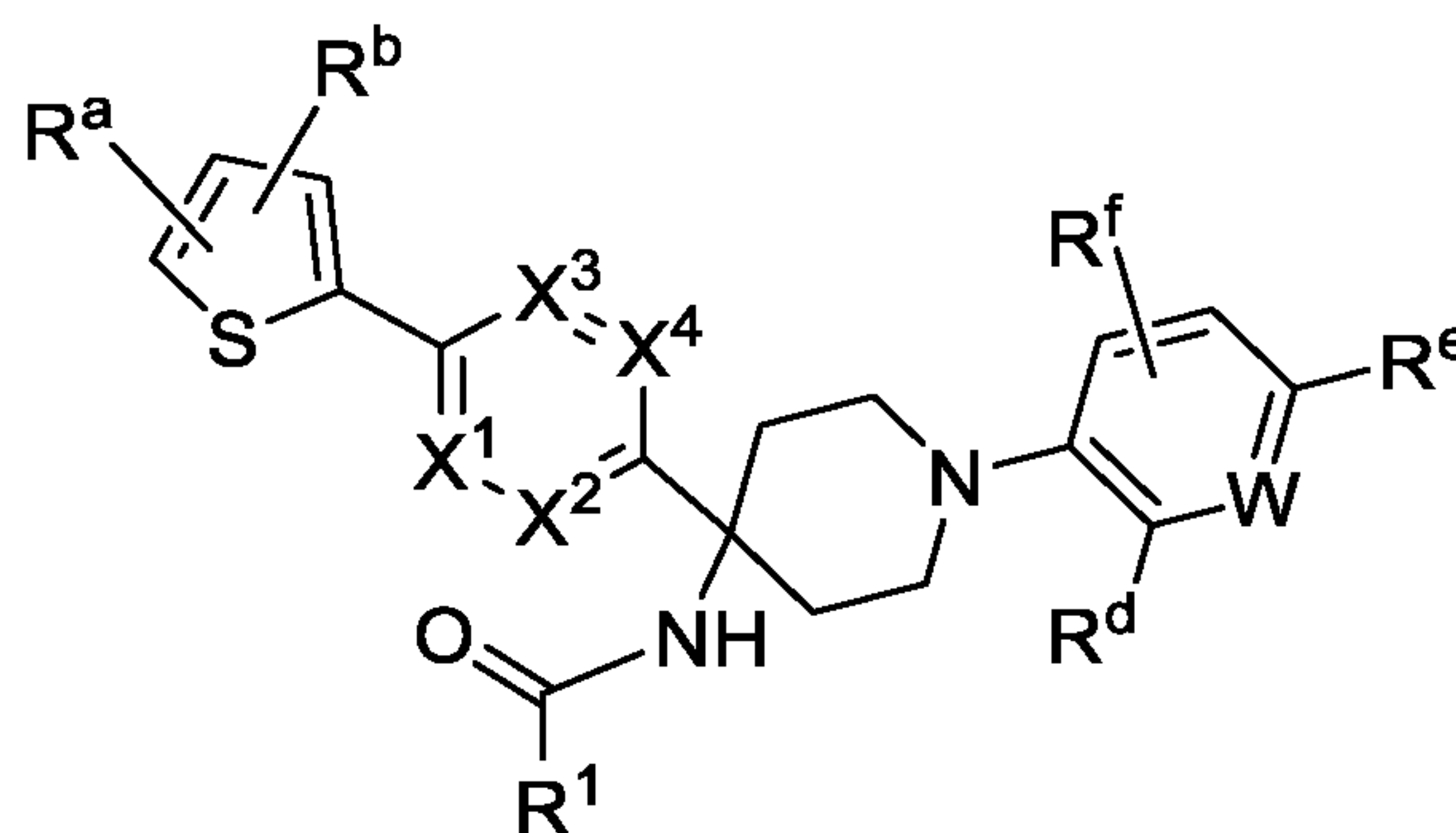
Formula (VIIf)
