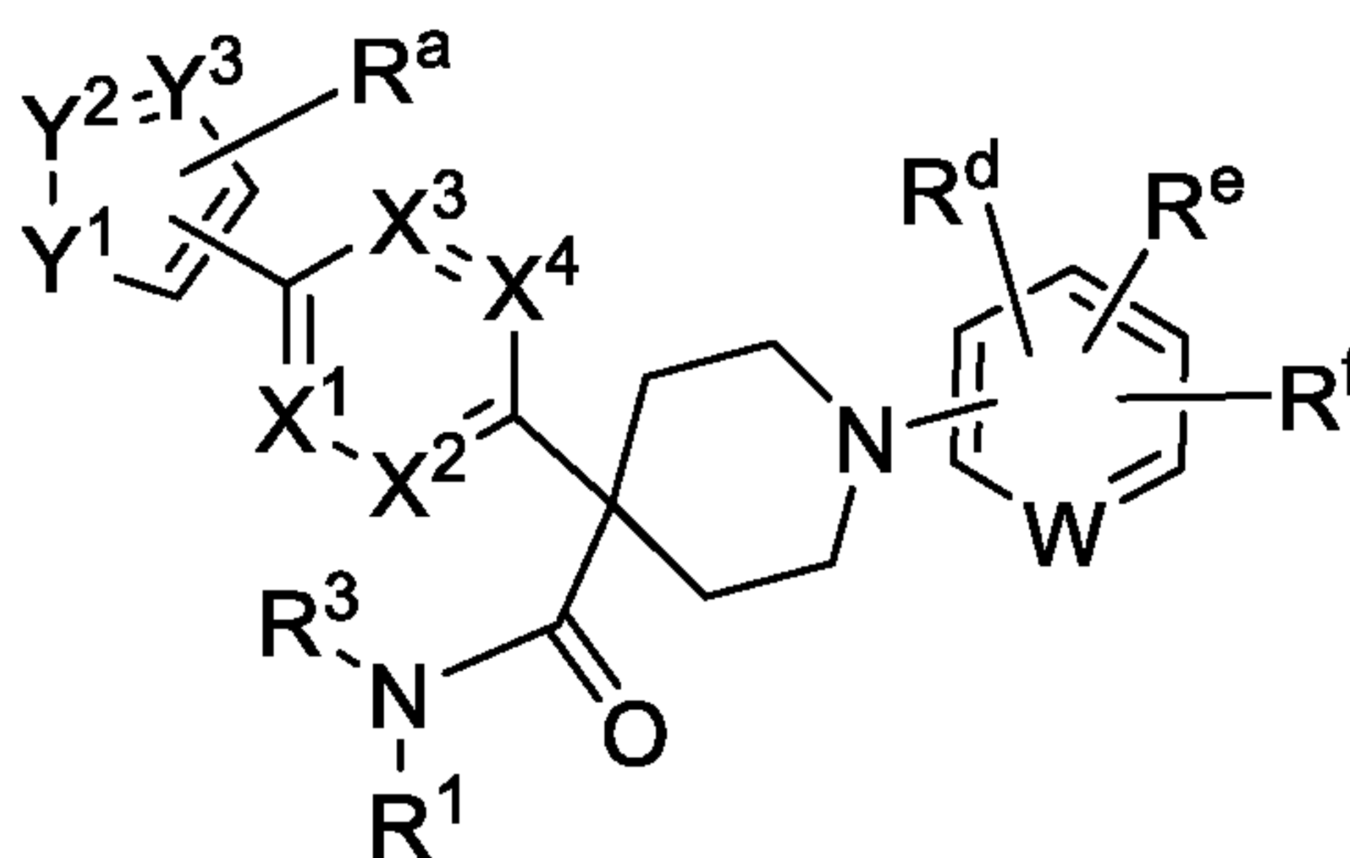
Formula (Va)
