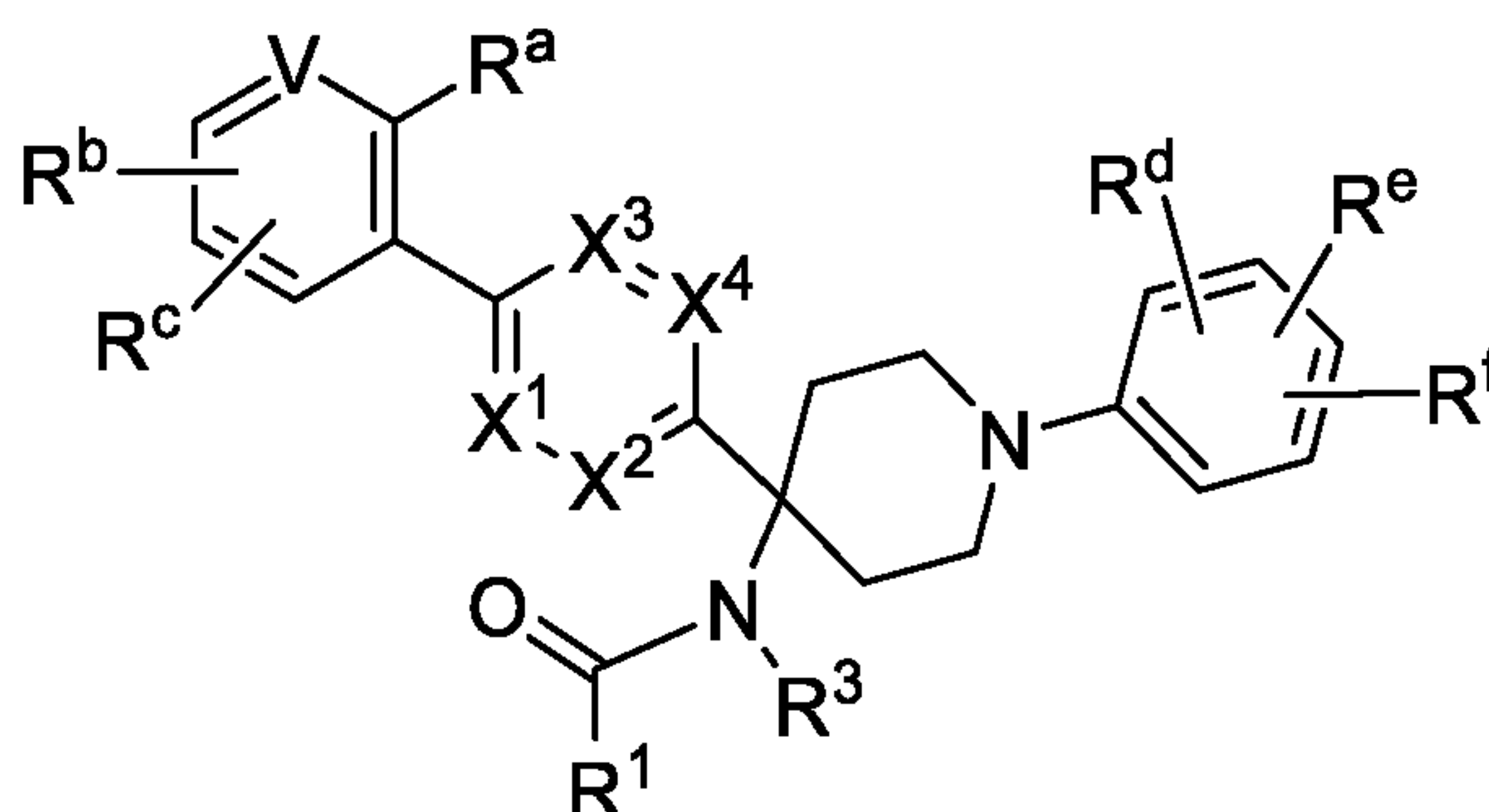
Formula (VIId)
