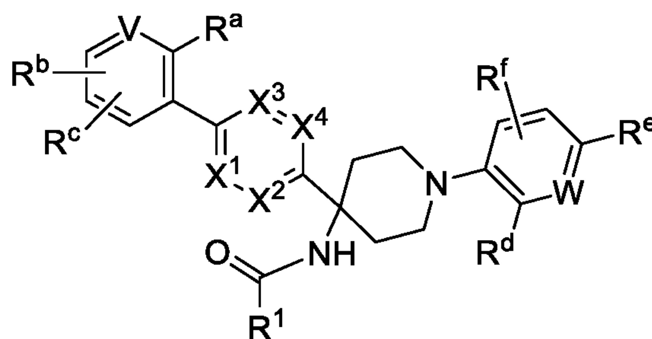
Formula (VIIe).
