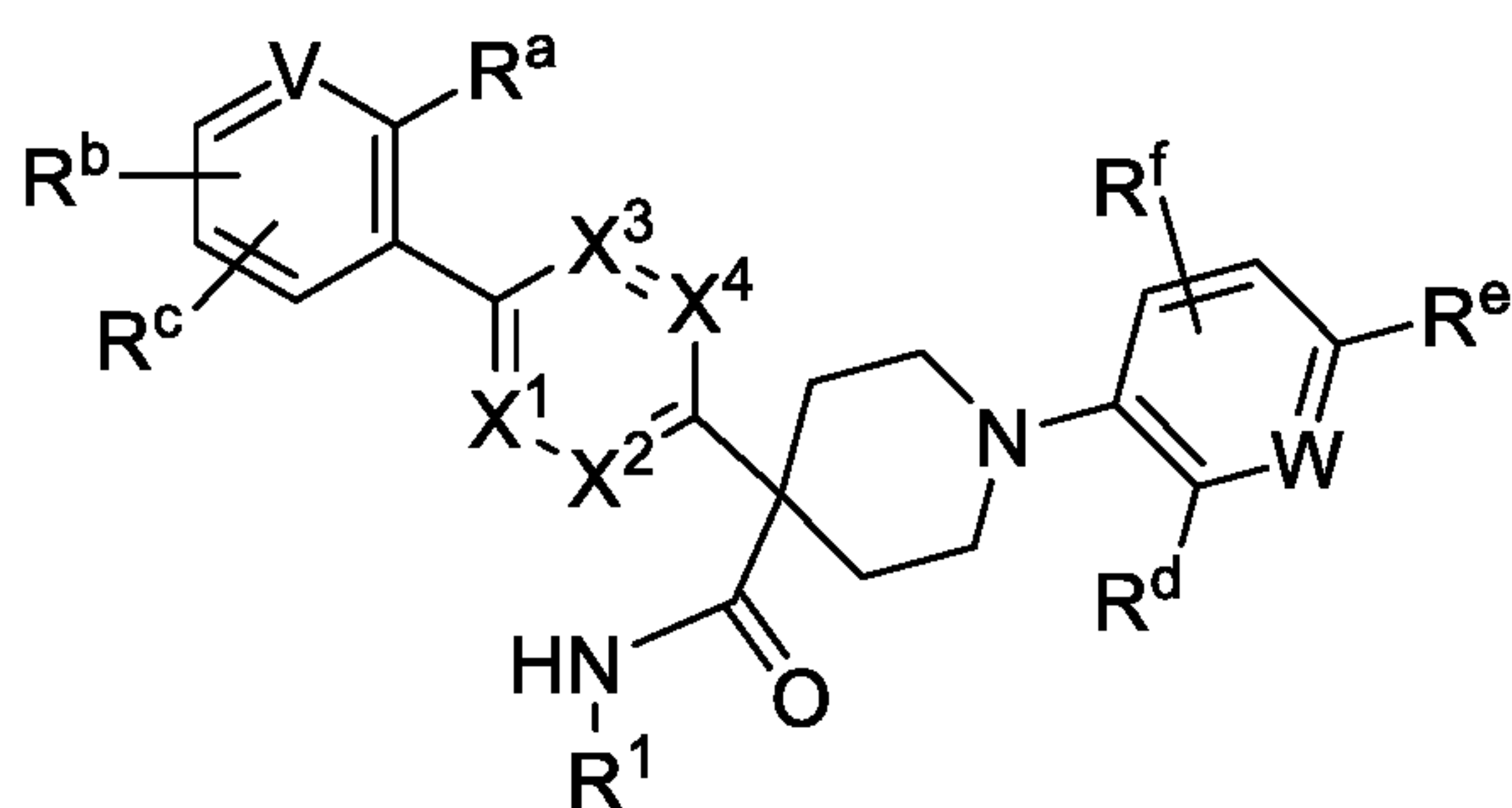
Formula (VIIb)
