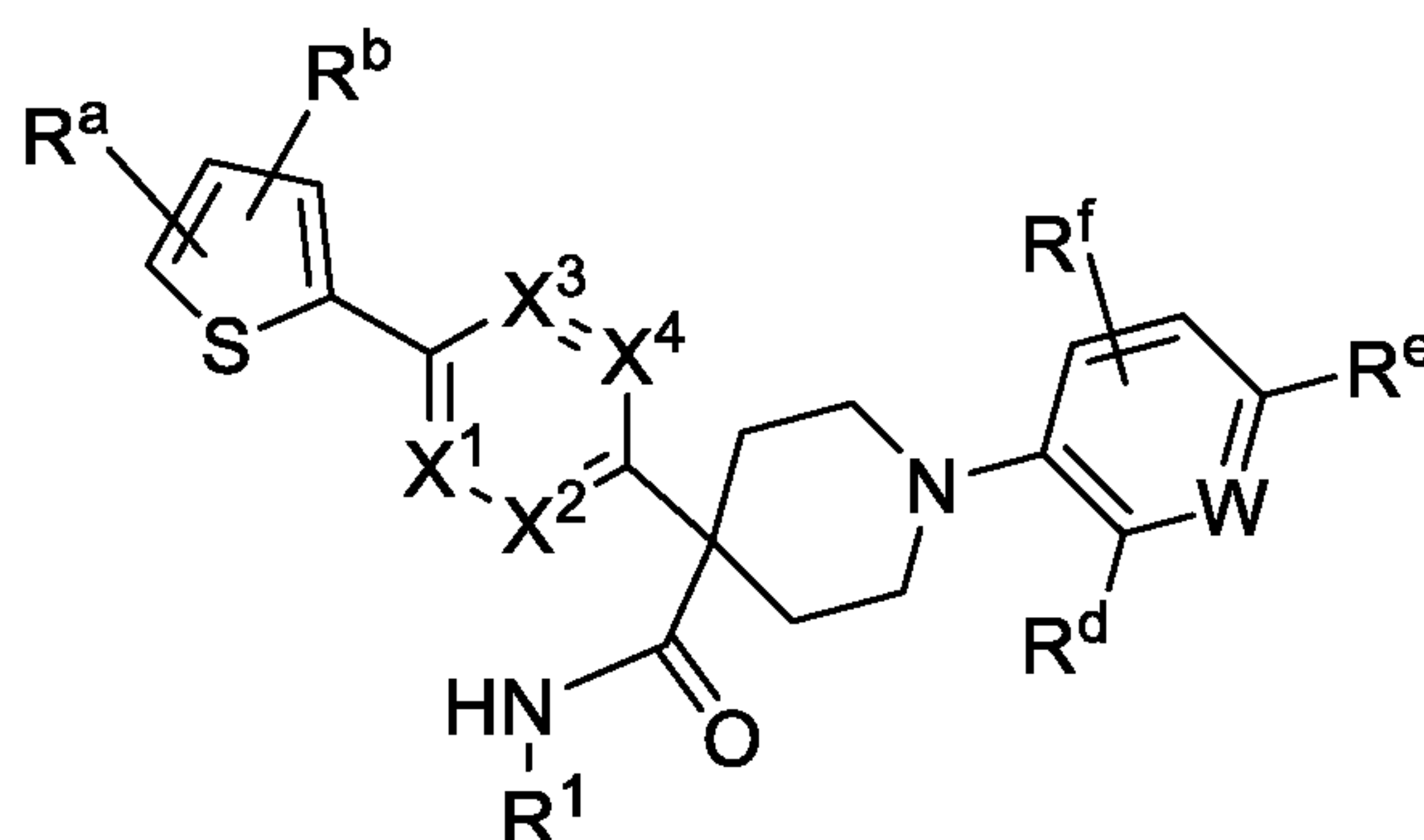
Formula (VIIf)
