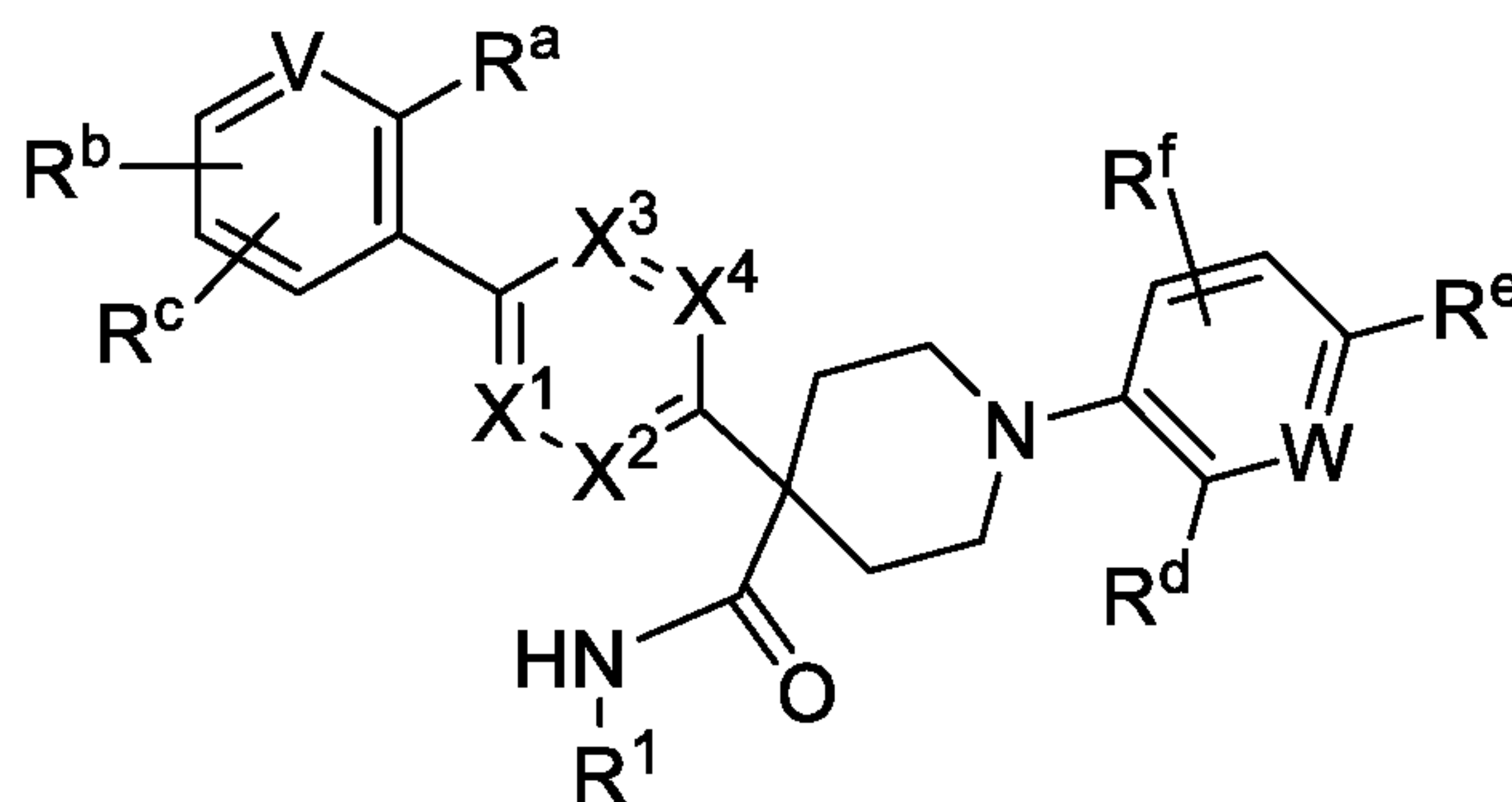
Formula (VIIb)
