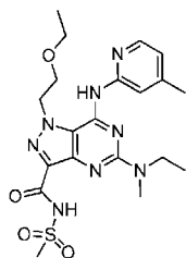
1-(2-ethoxyethyl)-5-(ethyl(methyl)amino)-7-((4-methylpyridin-2-yl)amino)-N-(methylsulfonyl)-1H-pyrazolo[4,3-d]pyrimidine-3-carboxamide
