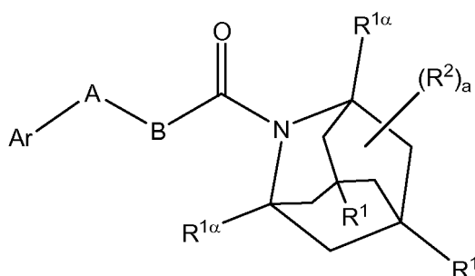
Formule (I)
