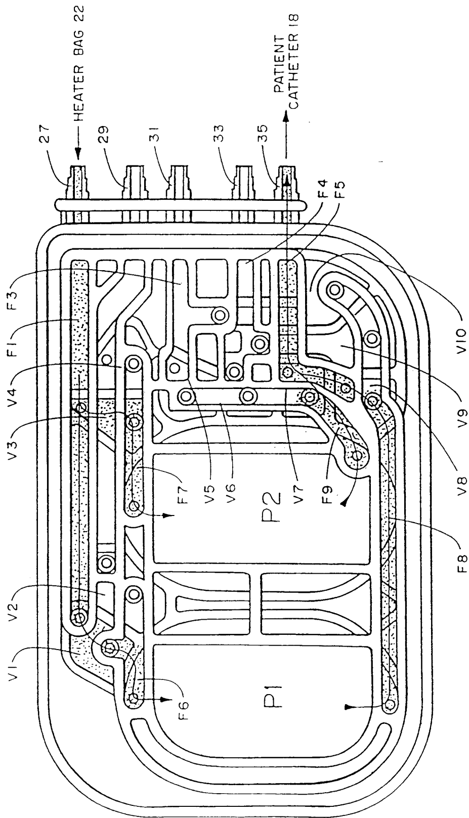
FIG. 32 (FILL)
