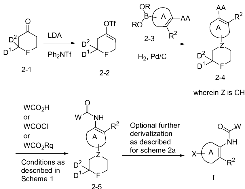
Scheme 2a
