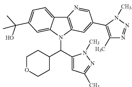
Enantiomer A
