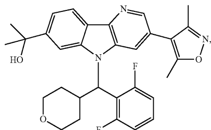
Enantiomer A
