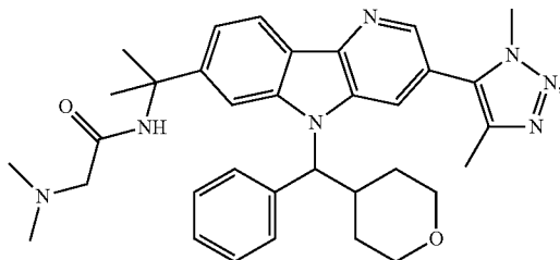
Enantiomer B
