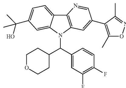
Enantiomer B
