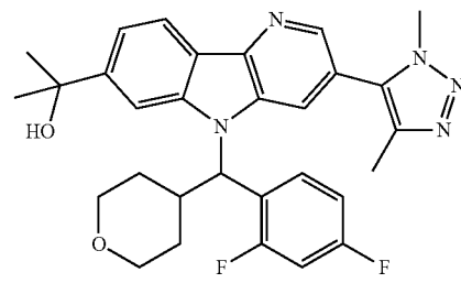
Enantiomer B
