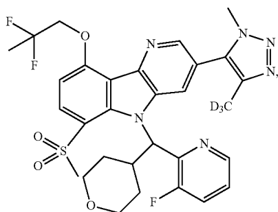
Enantiomer A
