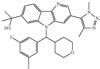
Enantiomer B
