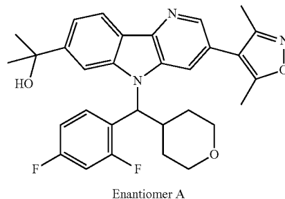
Enantiomer A
