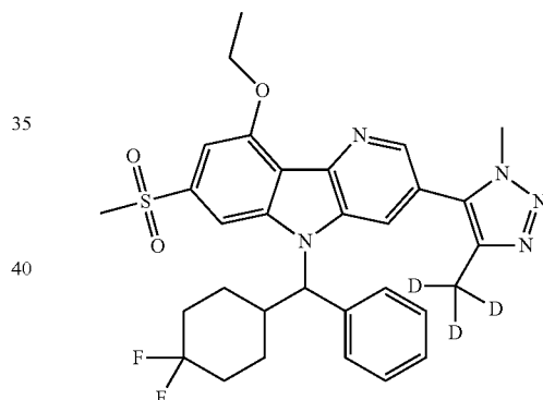
Enantiomer A
