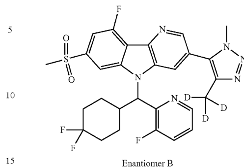
Enantiomer B
