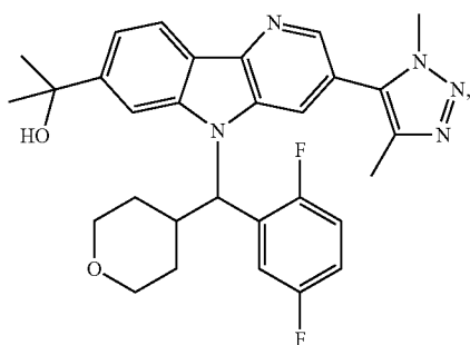
Enantiomer A
