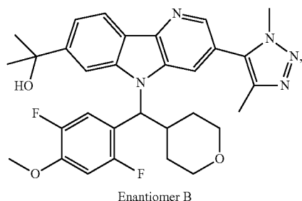
Enantiomer B
