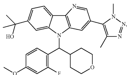
Enantiomer B
