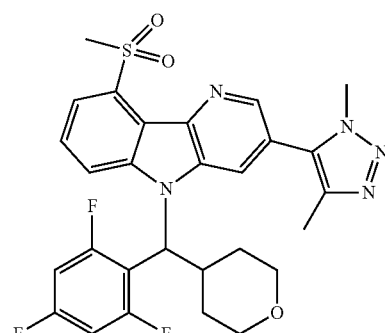
Enantiomer A
