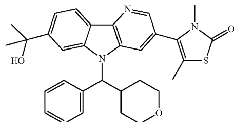
Enantiomer A
