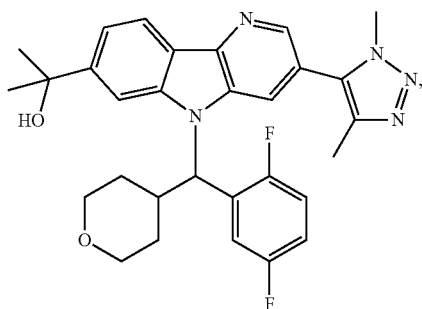
Enantiomer B
