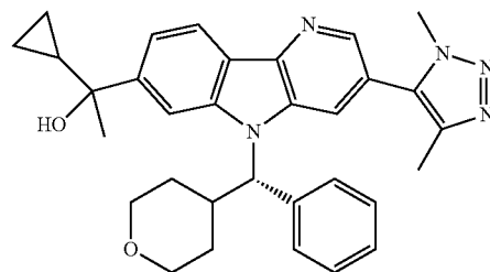
Enantiomer B
