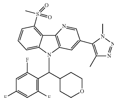
Enantiomer B
