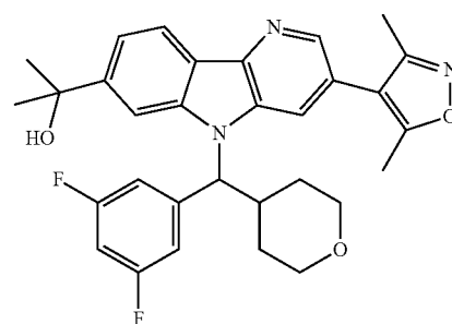
Enantiomer B
