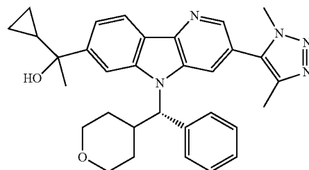
Enantiomer A
