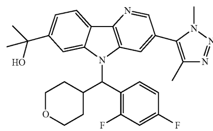
Enantiomer A
