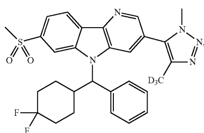
Enantiomer A
