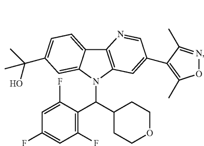
Enantiomer A
