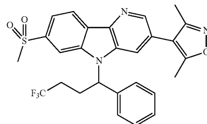
Enantiomer B
