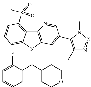
Enantiomer A
