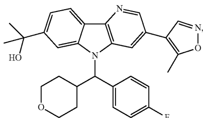
Enantiomer A
