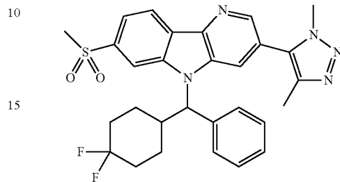
Enantiomer A
