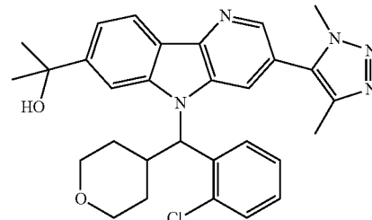
Enantiomer B
