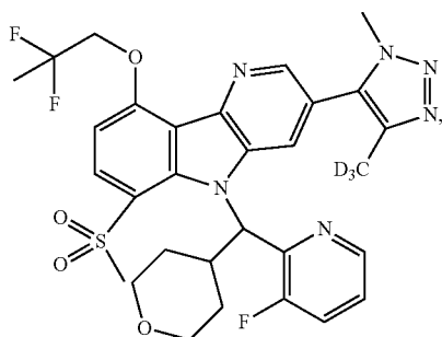
Enantiomer B
