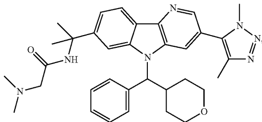
Enantiomer A
