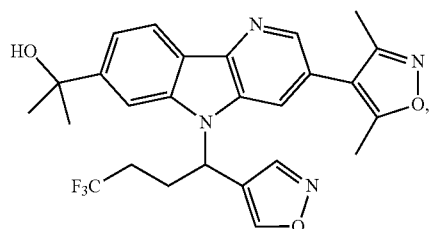
Enantiomer B
