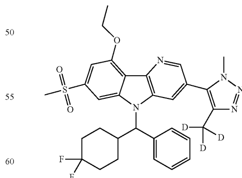
Enantiomer B
