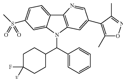
Enantiomer B
