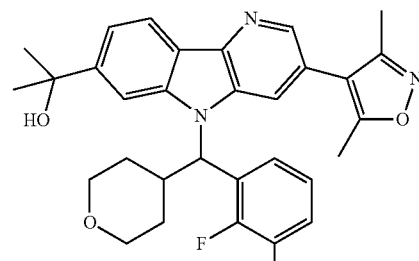
Enantiomer A
