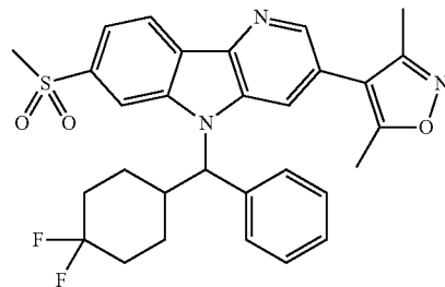
Enantiomer A
