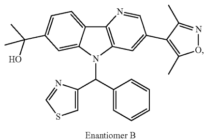
Enantiomer B
