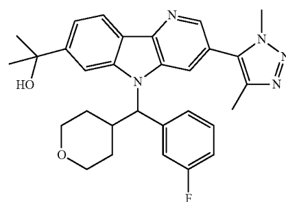
Enantiomer A
