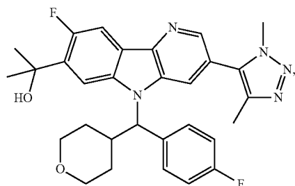
Enantiomer A
