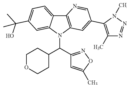
Enantiomer A
