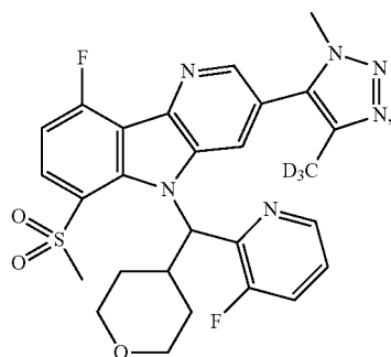
Enantiomer A
