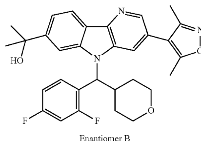
Enantiomer B
