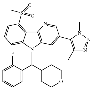
Enantiomer B
