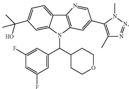
Enantiomer A
