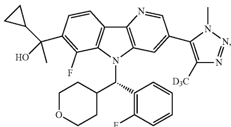
Enantiomer A
