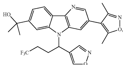
Enantiomer A
