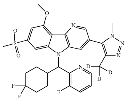
Enantiomer B
