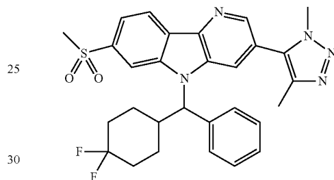
Enantiomer B
