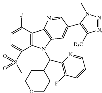
Enantiomer B
