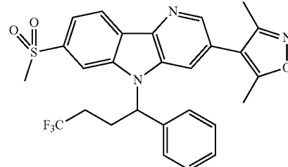
Enantiomer A
