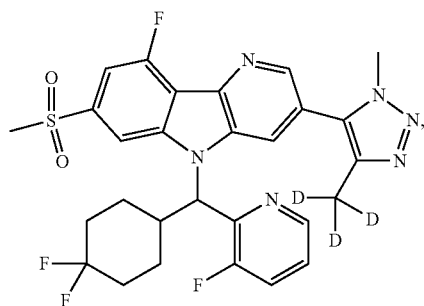
Enantiomer A
