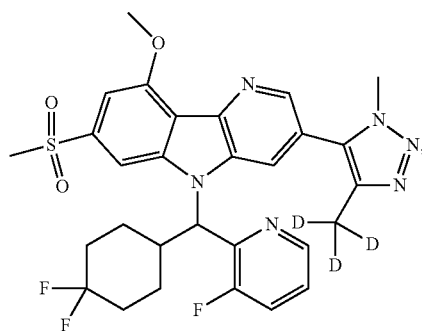
Enantiomer A
