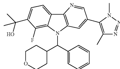
Enantiomer A
