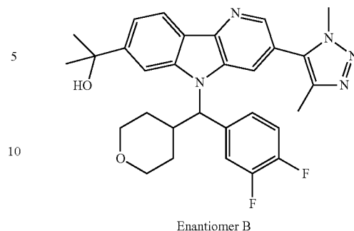
Enantiomer B
