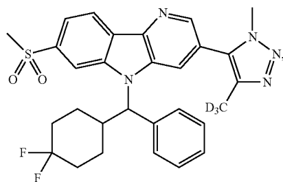
Enantiomer B
