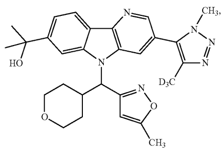
Enantiomer A
