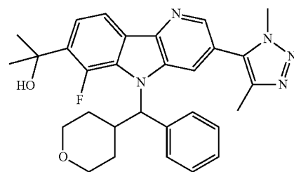
Enantiomer B
