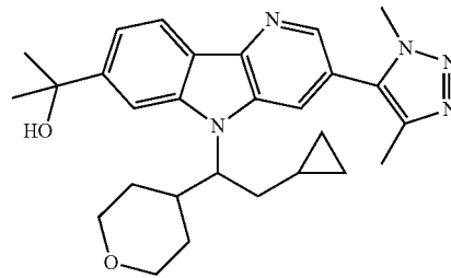
Enantiomer A
