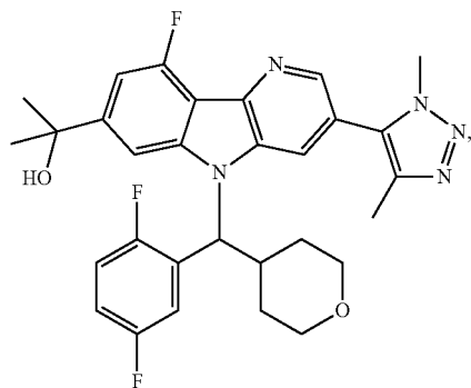
Enantiomer A
