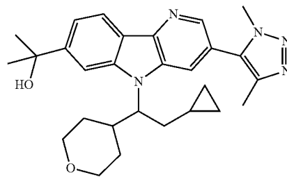
Enantiomer B
