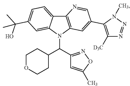
Enantiomer B
