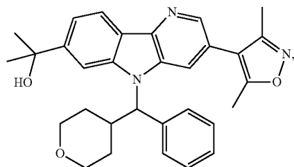
Enantiomer B
