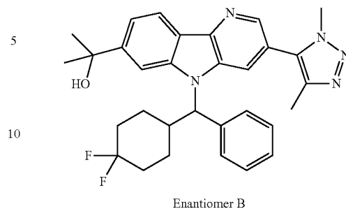
Enantiomer B
