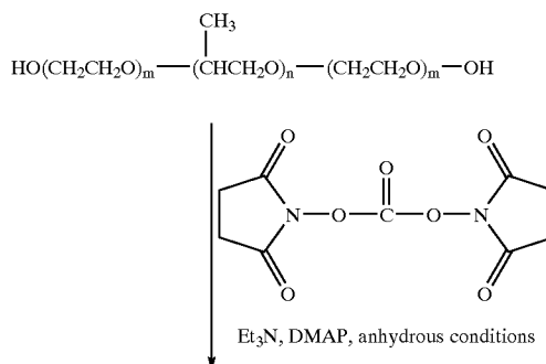
SCHEME 1a
