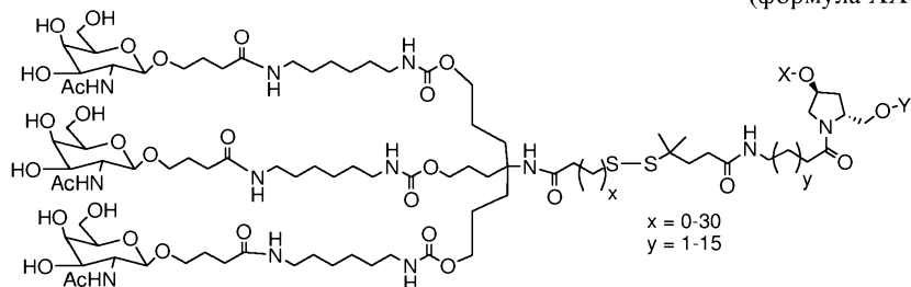
(формула XXVIII),
