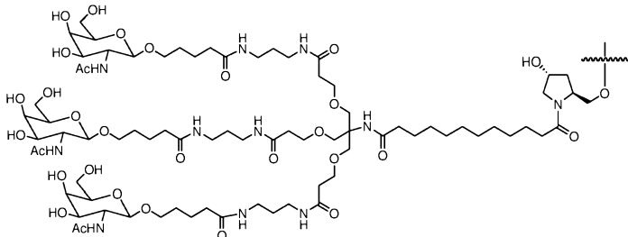
(формула XXV),
