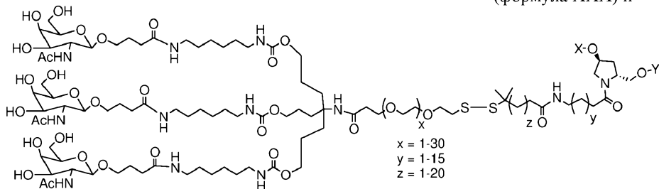
(формула XXXI),
