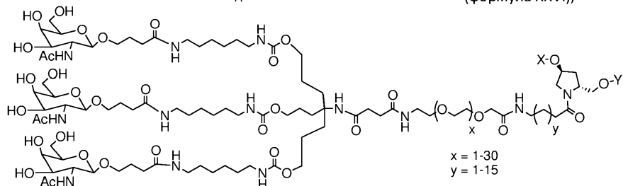
(формула XXVII),
