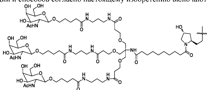
(формула XXIV),
