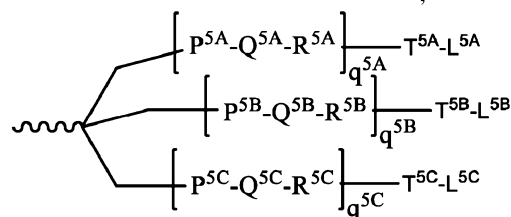
формула XXXV
