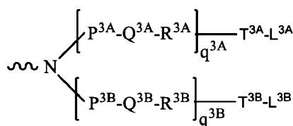
формула XXXIII
