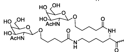
, формула XIV,
