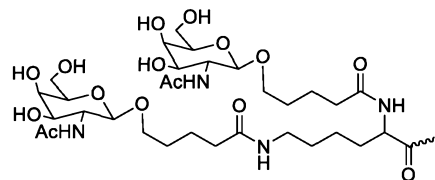
, формула XVI,
