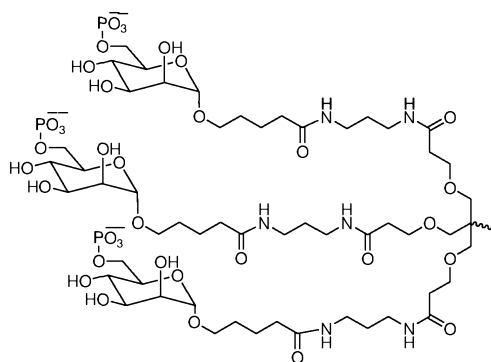
, формула XII,
