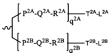
формула XXXII
