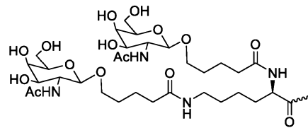
, формула XV,
