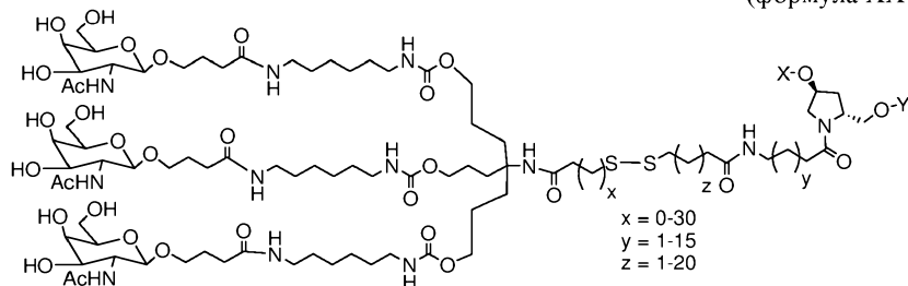
(формула XXIX),
