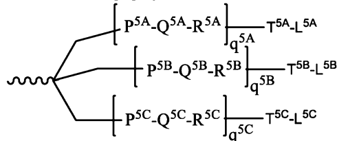
формула XXXV
