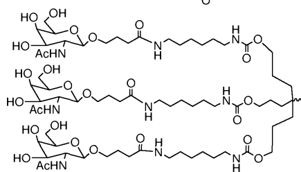
, формула XIII,
