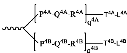
формула XXXIV
