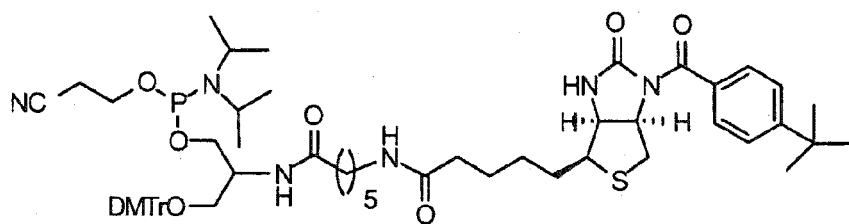
Biotin-Serinol Amidite
