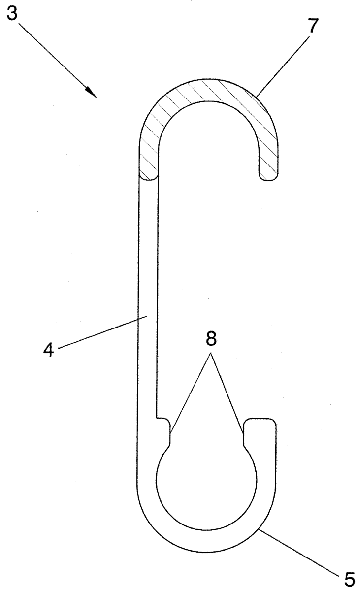
A - A FIG. 4
