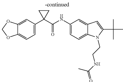
N-(1-(2-Acetamidoethyl)-2-tert-butyl-1H-indol-5-yl)-1-(benzo[d][1,3]-dioxol-5-yl)cyclopropanecarboxamide
