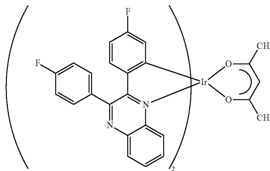
Ir(Fdpq) 2 (acac)
