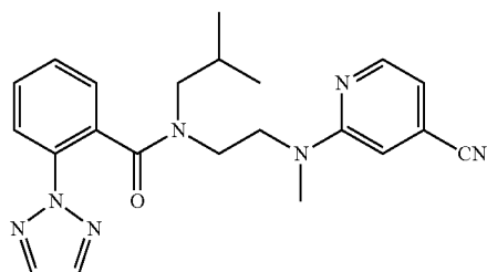
N-(2-((4-cyanopyridin-2-yl)(methyl)amino)ethyl)-N-isobutyl-2-(2H-1,2,3-triazol-2-yl)benzamide (Example G-8)
