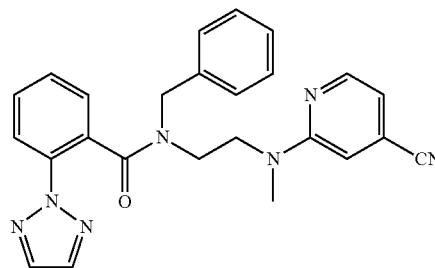
N-benzyl-N-(2-((4-cyanopyridin-2-yl)(methyl)amino)ethyl)-2-(2H-1,2,3-triazol-2-yl)benzamide (Example G-6)
