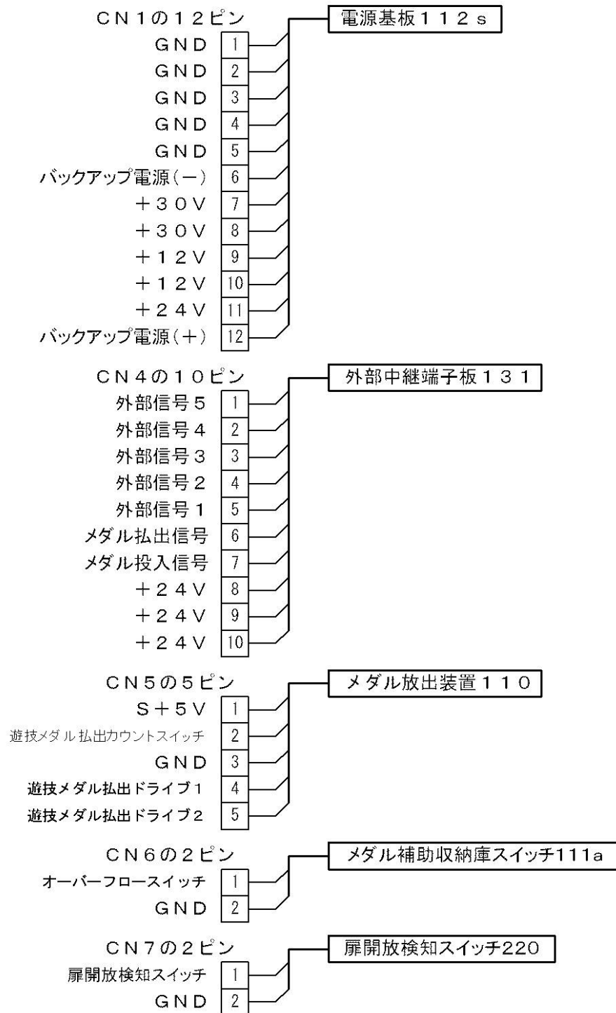
主中継基板 1 2 2
