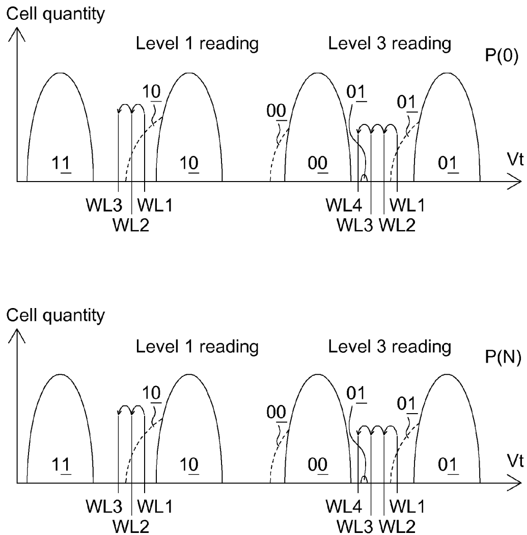
FIG. 6B(PRIOR ART)
