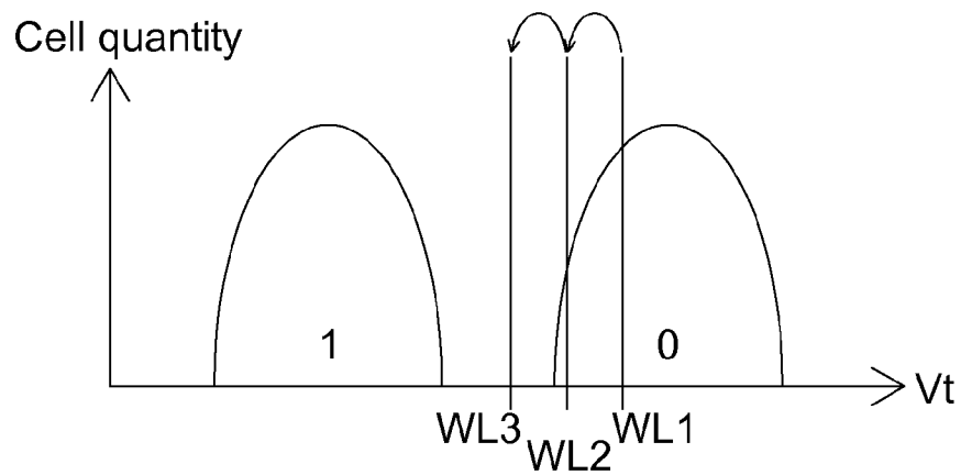
FIG. 2B(PRIOR ART)
