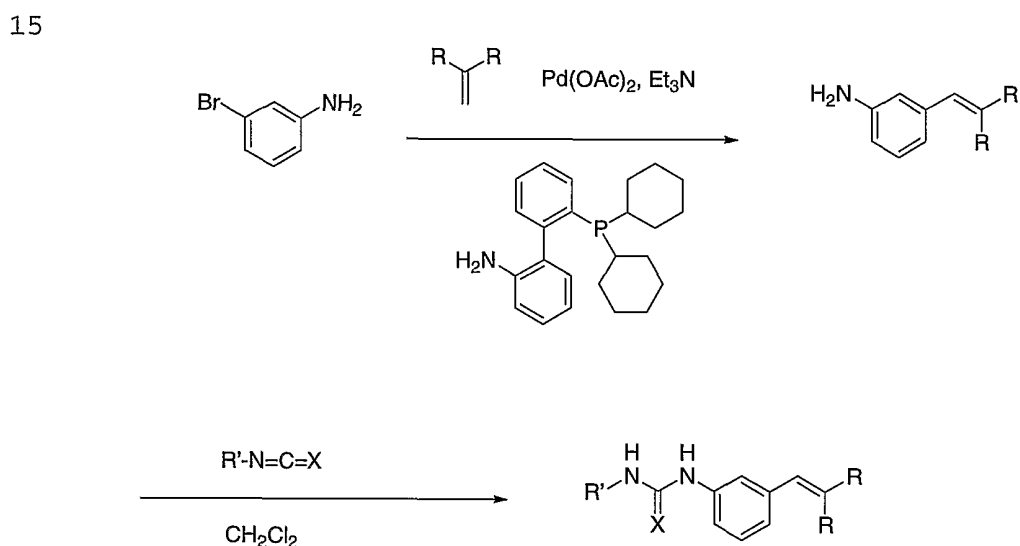
Scheme VI
