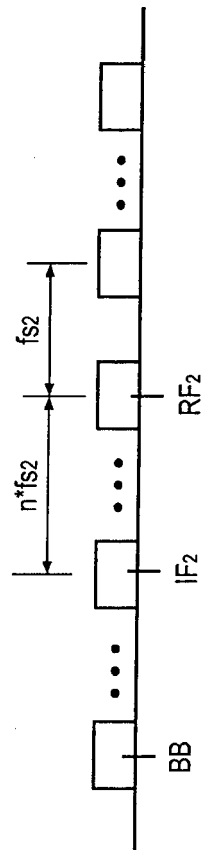
FIG. 108 S&H output 2 412
