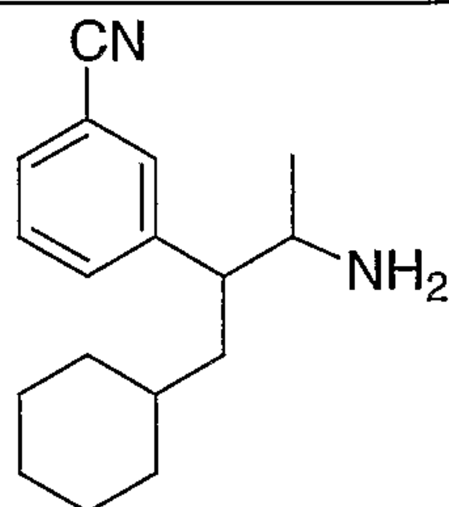
2-(3-Cyanophenyl)-3-cyclohexyl-1-methylpropylamine
