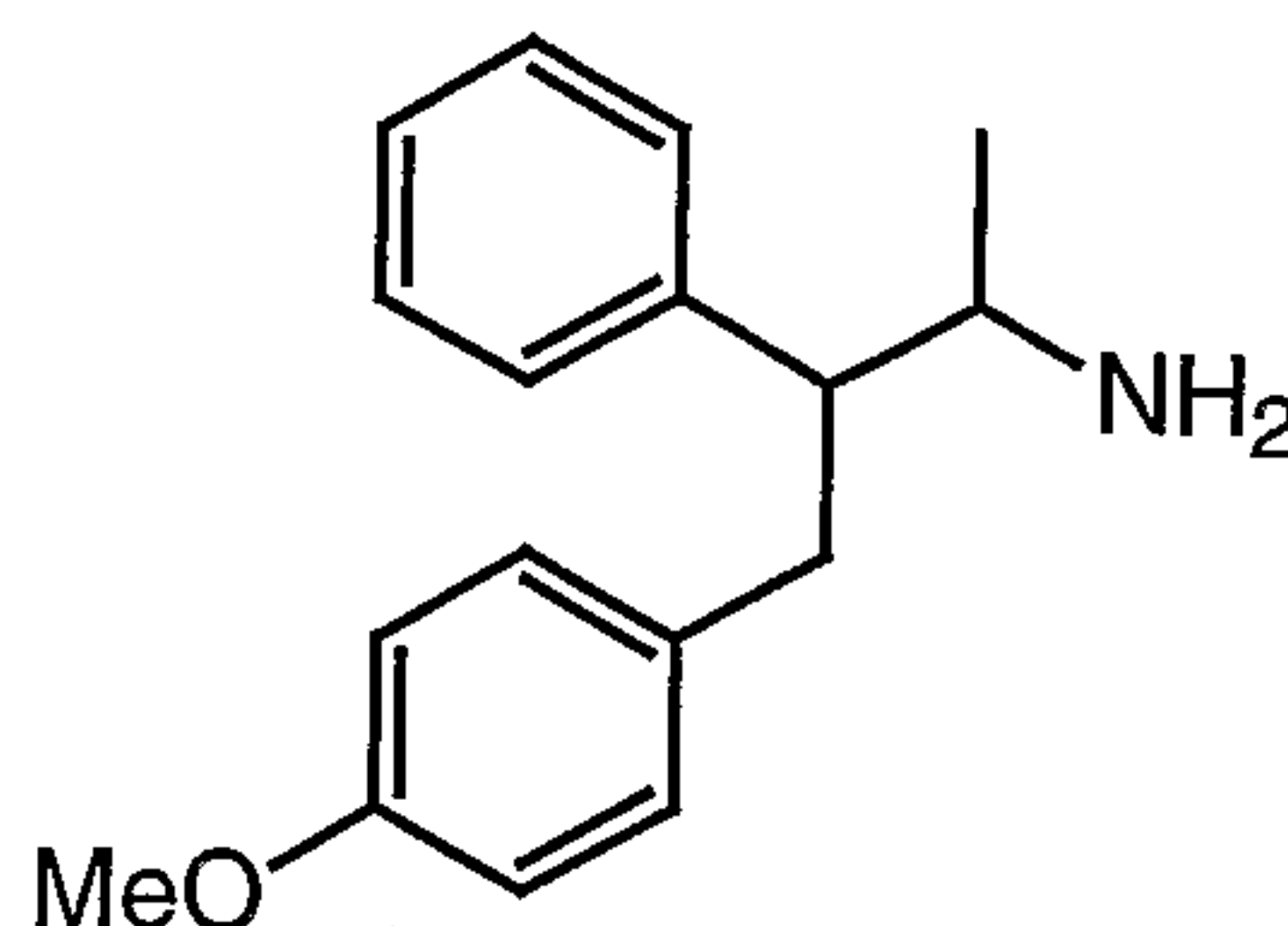
4-(4-Methoxyphenyl)-3-phenylbutan-2-amine
