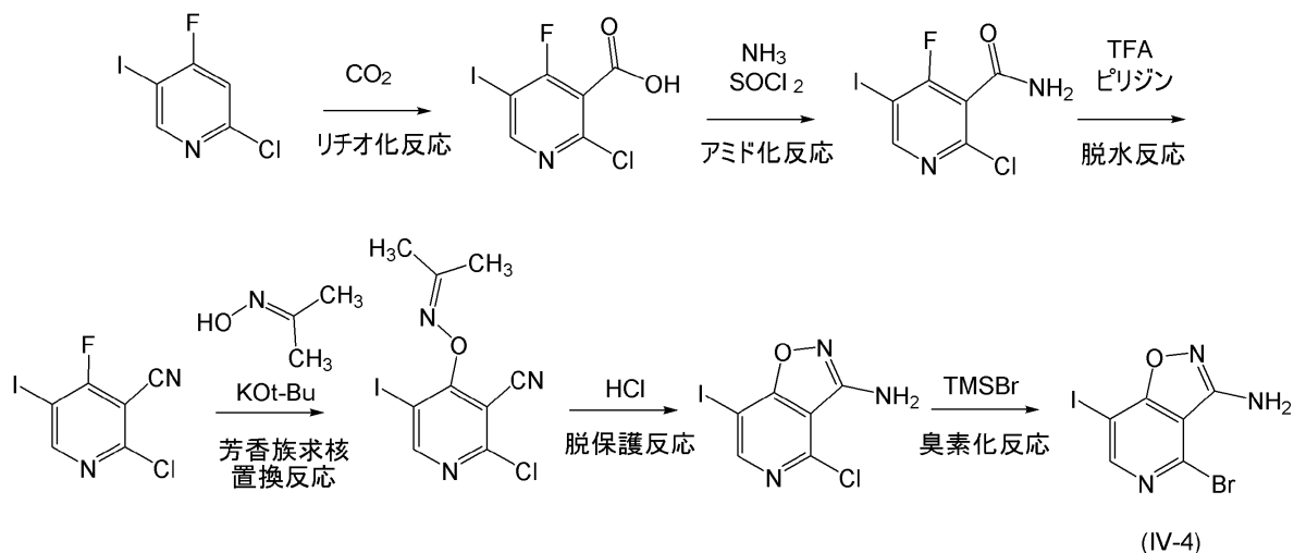
反応工程式 2
