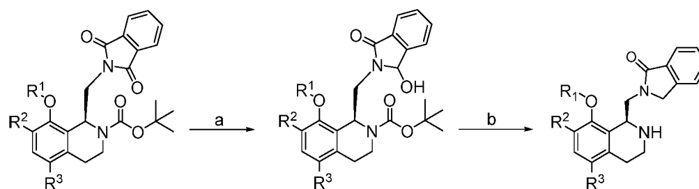
Scheme 4: a) NaBH 4 , MeOH; b) TFA, Et 3 SiH.
