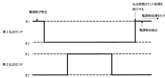
＜払出センサの作用図 ボタンA＞
