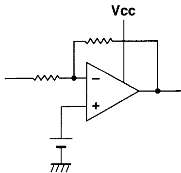
INVERTING AMPLIFIER Q1
