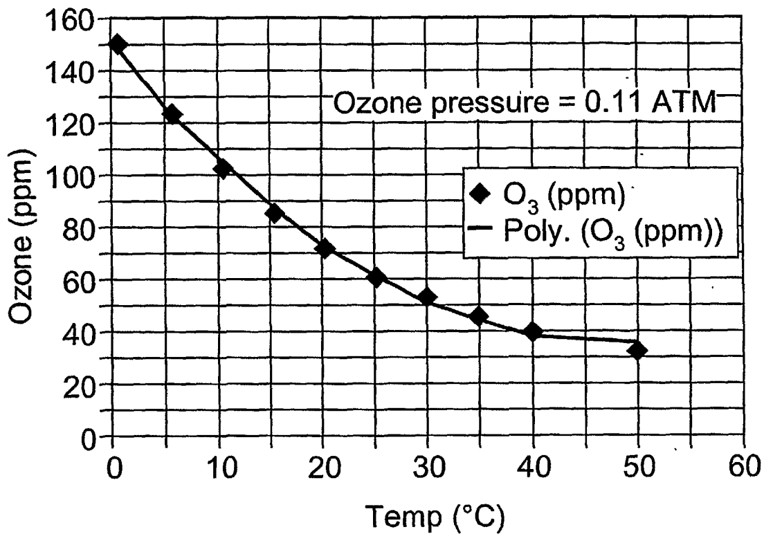
O 3 (ppm) vs DI Temp
