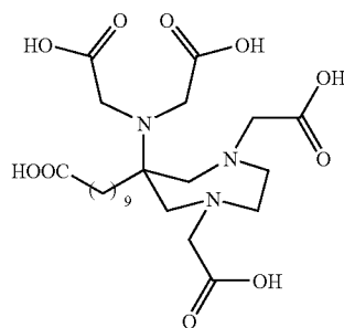
ω-CarboxydecylAAZTA
