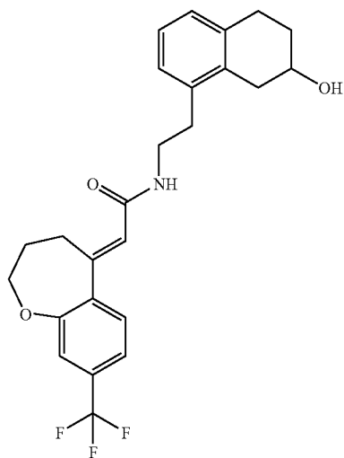
EXAMPLE 223
