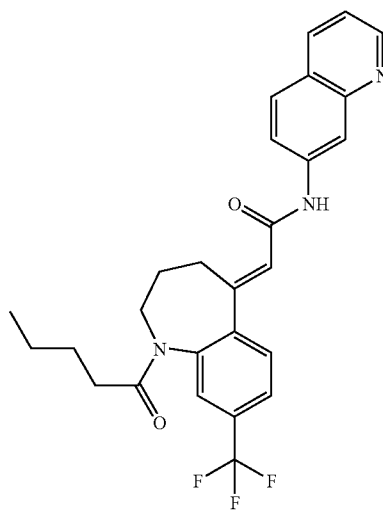
EXAMPLE 189
