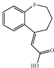
Formula (4) RN = 14861-92-8
