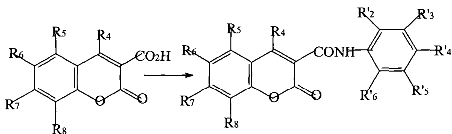
(IIb)
