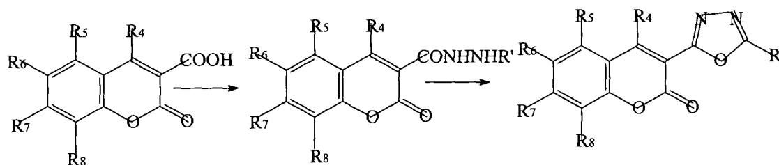
(IIIf)
