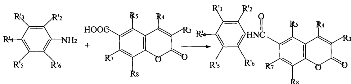
(IIId)
