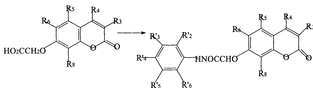
(IIe)
