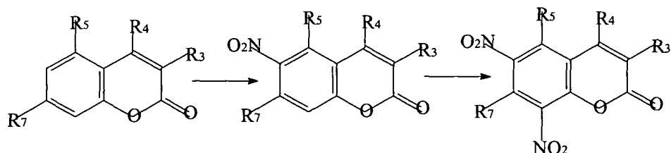
(IIa)
