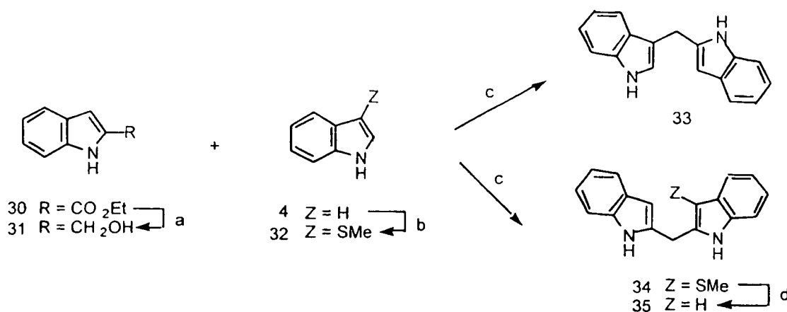
Scheme IV. a. \text{LiAlH}_4 . b. NCS, (\text{CH}_3)_2\text{S} , \text{CH}_2\text{Cl}_2 ; Xylenes, reflux. c. (\text{CF}_3\text{SO}_3)_3\text{Sc} . d. Raney Ni, EtOH.
