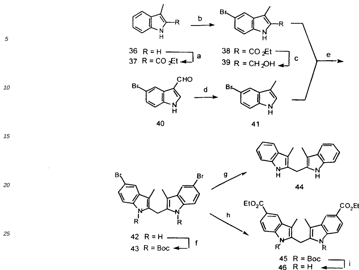
Scheme V. a. n -BuLi, CO 2 ; t -BuLi, ClCO 2 CH 2 CH 3 . b. NBS. c. LiAlH 4 . d. LiAlH 4 , 60°C. e. (CF 3 SO 3 ) 3 Sc. f. ( t -BuOCO) 2 O, DMAP. g. Raney Ni. h. t -BuLi; ClCO 2 CH 2 CH 3 . i. CF 3 CO 2 H.
