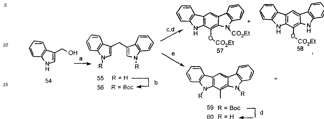
Scheme VII. a. aq. NaOH. b. (t\text{-BuOCO})_2\text{O} , DMAP. c. LiTMP; \text{ClCO}_2\text{CH}_2\text{CH}_3 . d. \text{CF}_3\text{CO}_2\text{H} . e. LTMP; (\text{CH}_3\text{CO})_2\text{O} .
