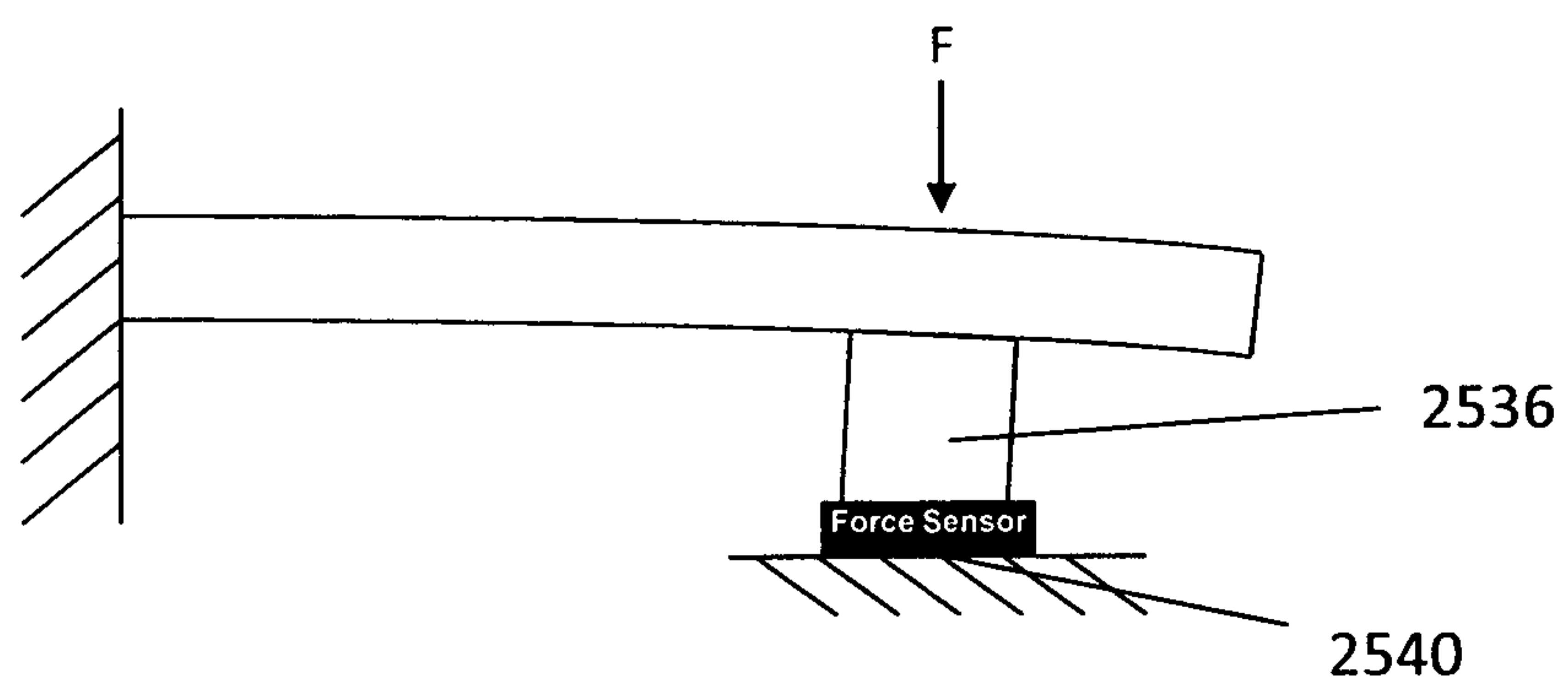
FIG. 25E
