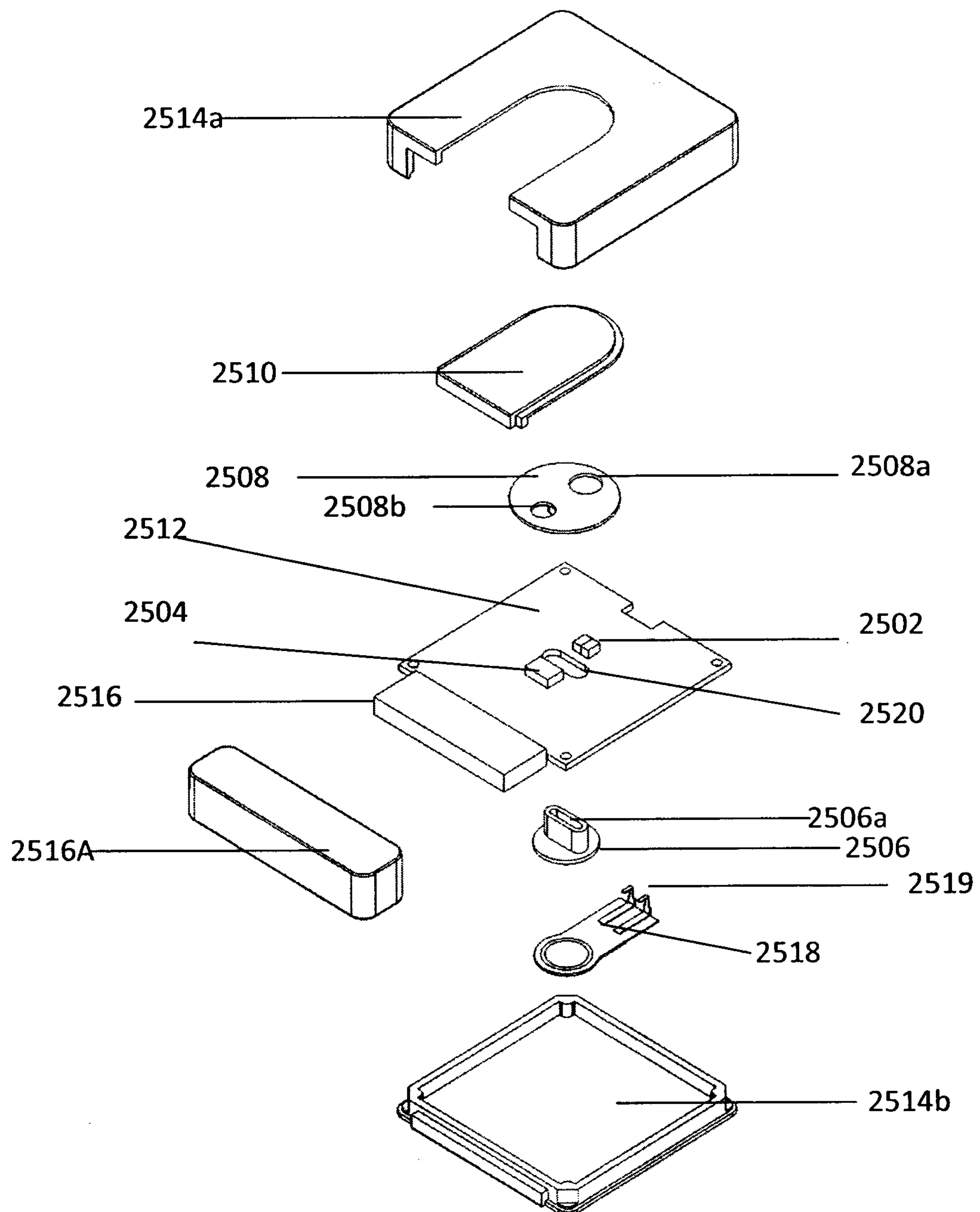
FIG. 25B
