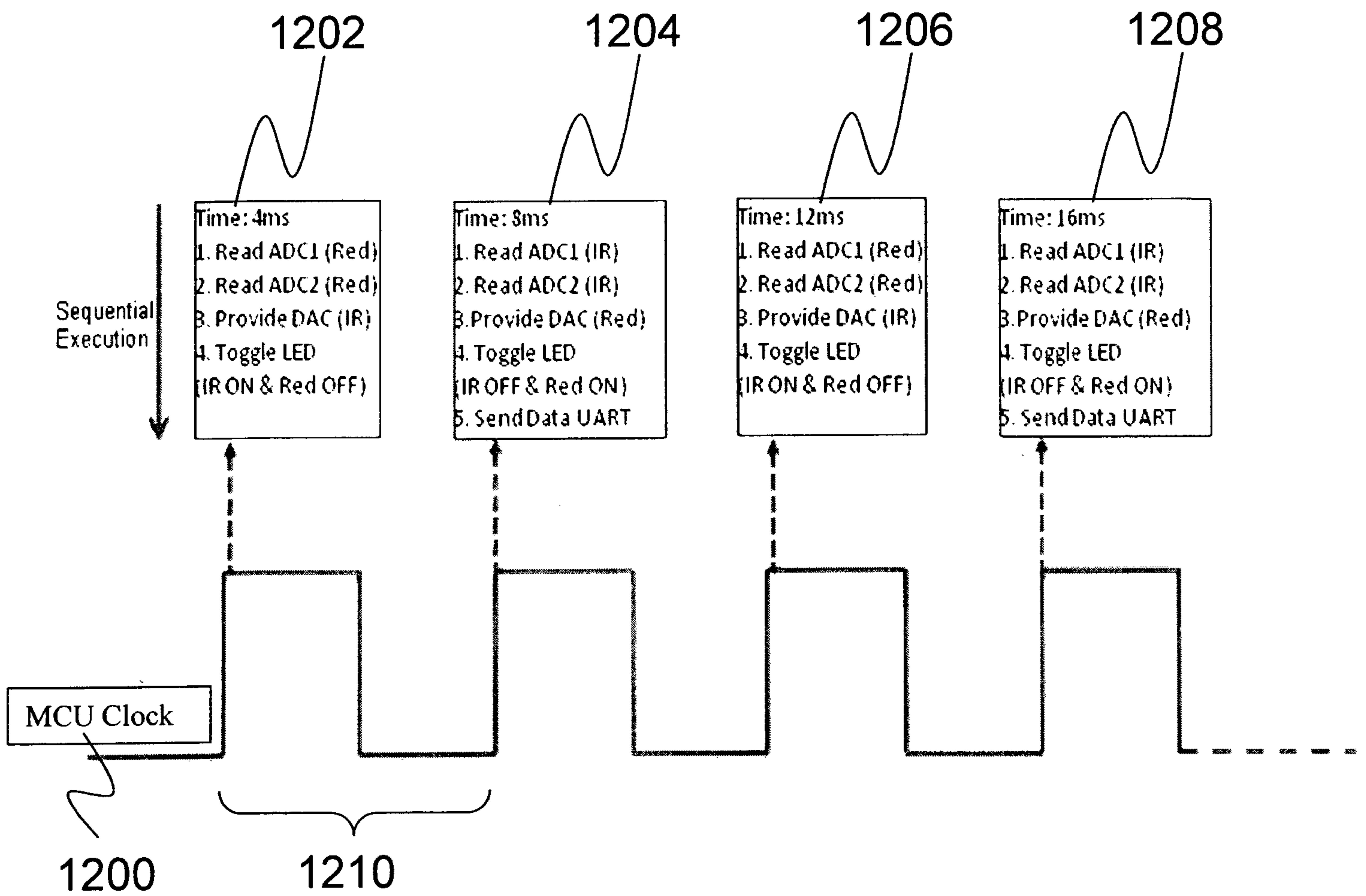
FIG. 19
