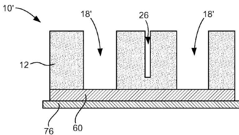
FIG. 21A
