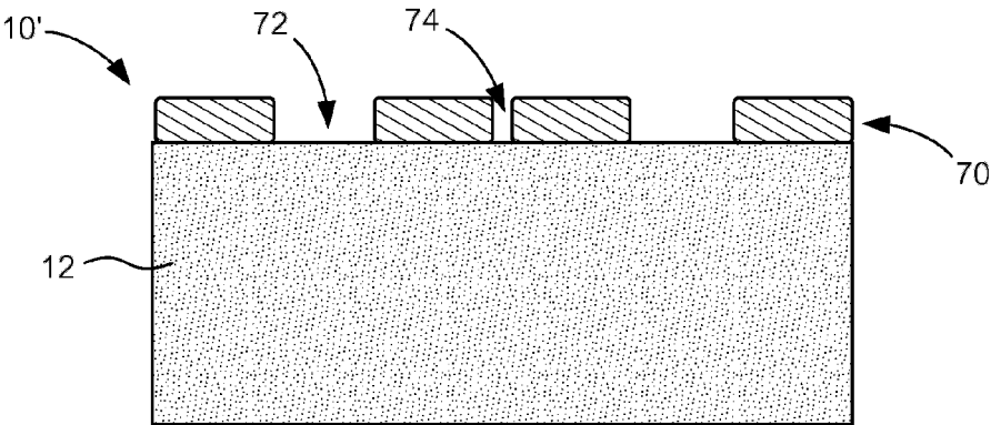
FIG. 20A
