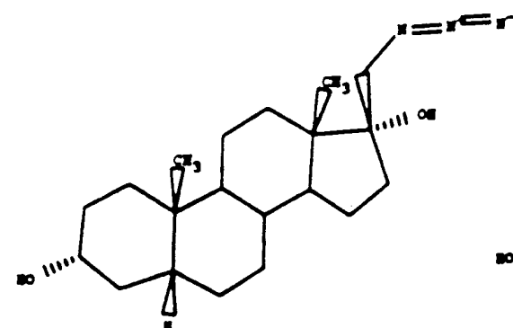
20-AZIDO-21-NOR-5 \beta -PREGNAN-3 \alpha , 17 \alpha -DIOL
