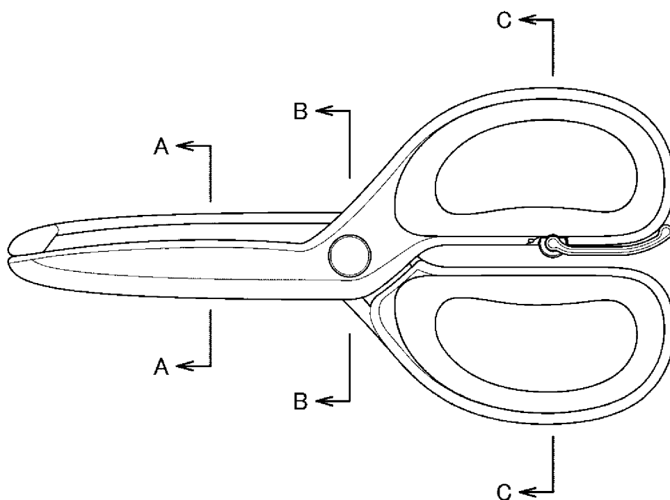
【前視圖】
