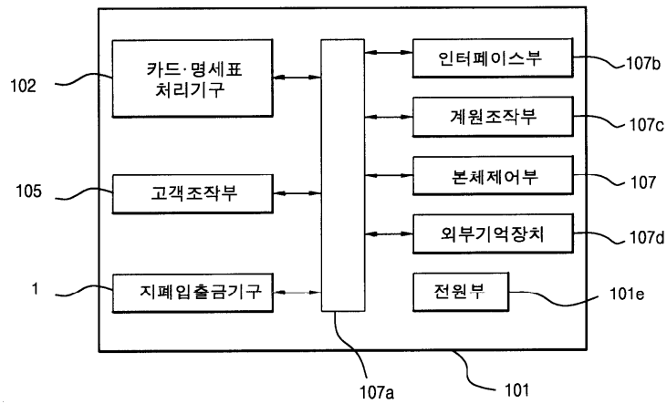
현금자동거래장치 (101)의 제어블럭도
