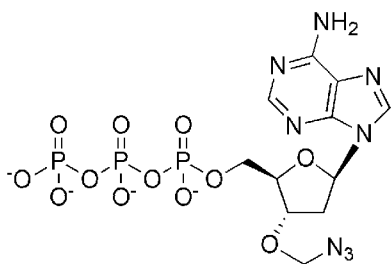
3'-O-N 3 -dATP
