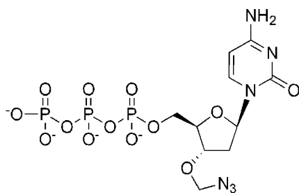
3'-O-N 3 -dCTP
