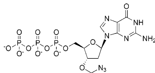
3'-O-N 3 -dGTP
