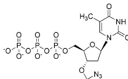
3'-O-N 3 -dTTP
