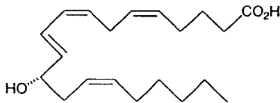
12(S)-HETE
