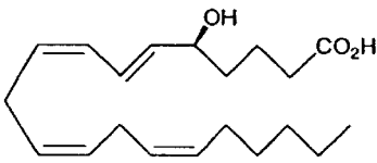
5(S)-HETE
