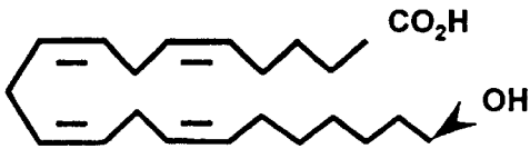
21-HETE
