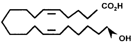
ps 20-HETE
