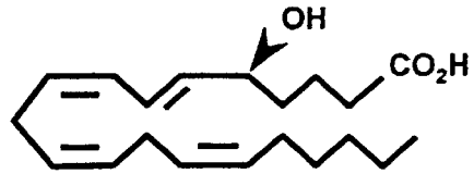
5(S)-HETE
