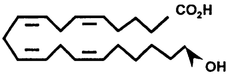
20-HETE
