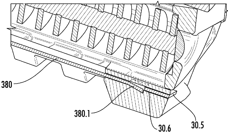
FIG. 19C
