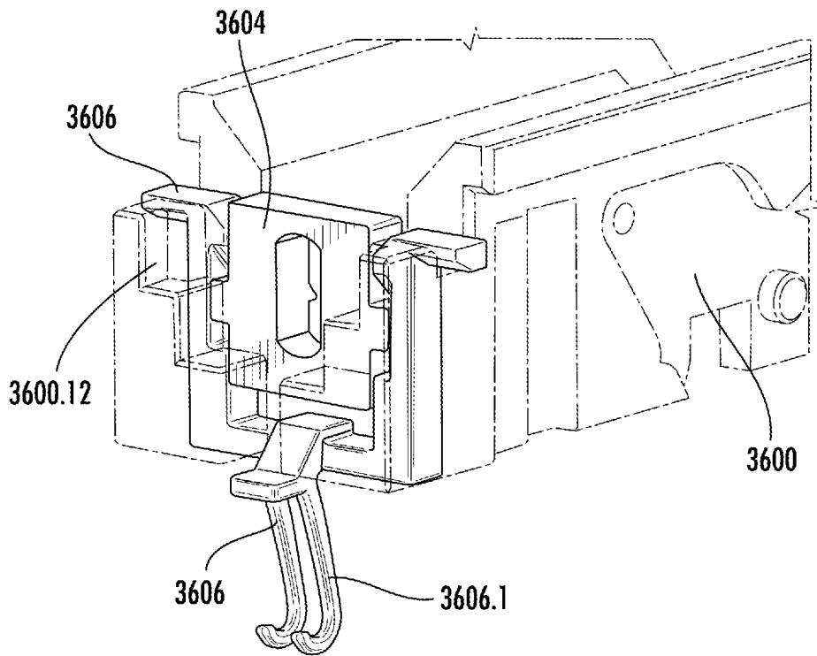
FIG. 17A
