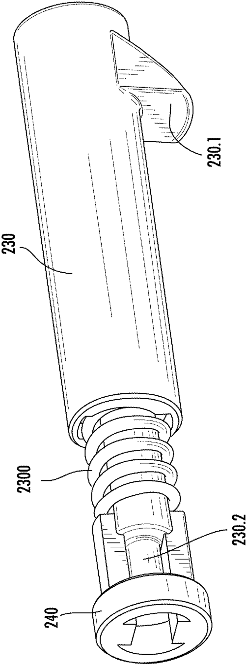
FIG. 15
