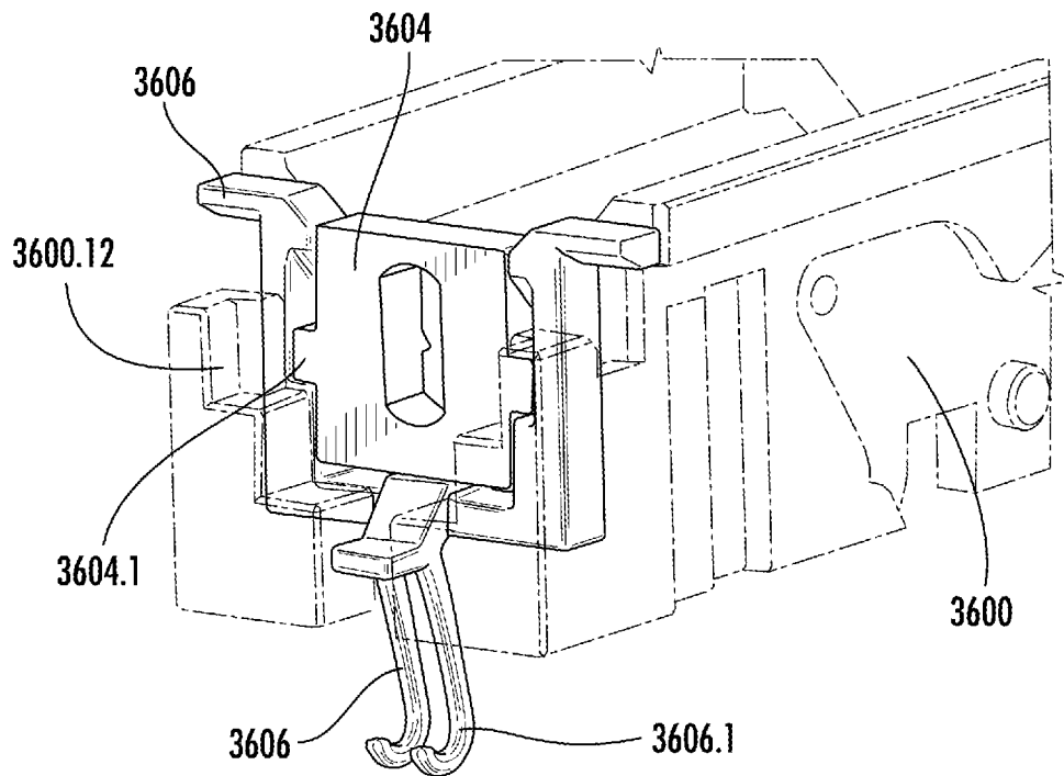
FIG. 17B
