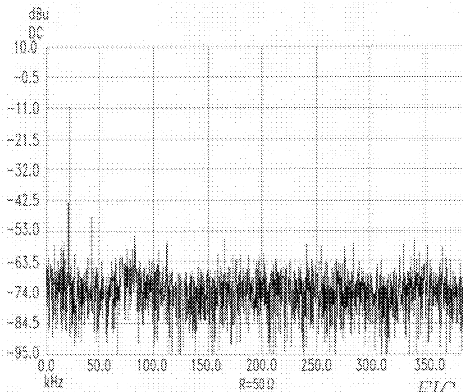
FIG. 9C
