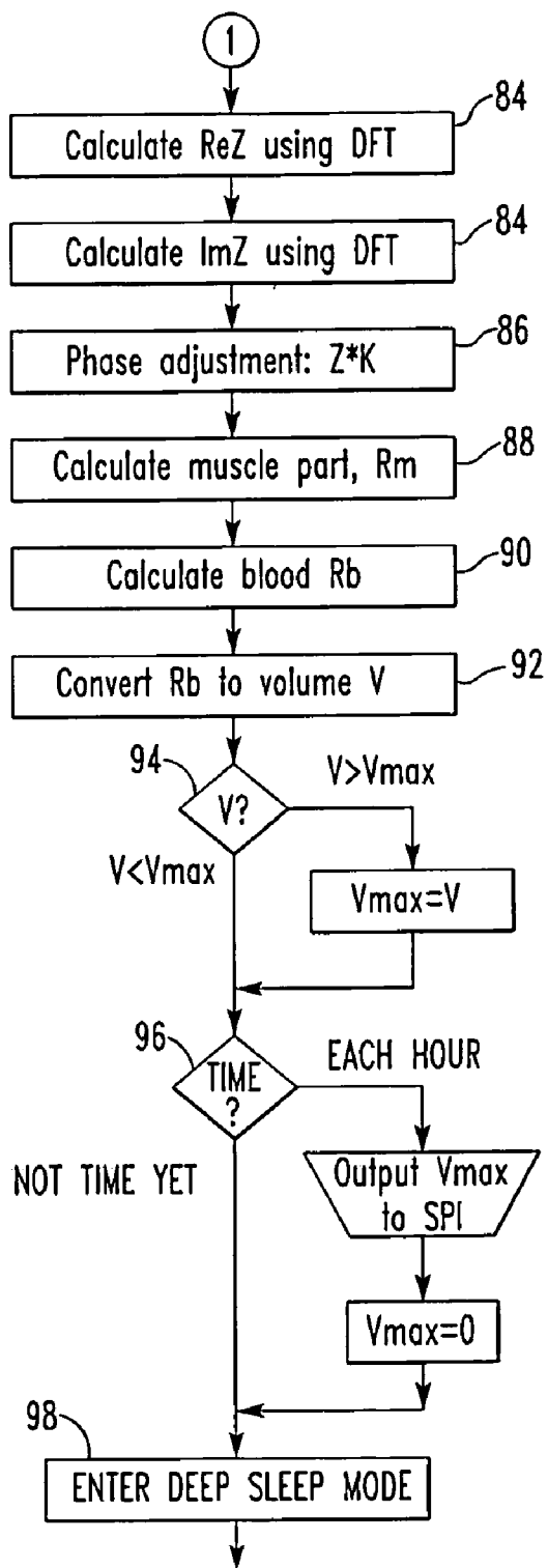
FIG.19B
