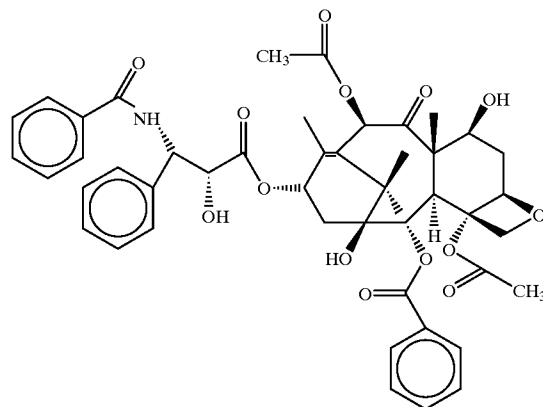
Paclitaxel
